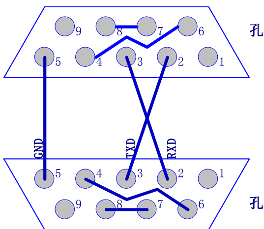
串行通讯电缆连线图
