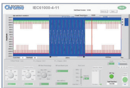
电压暂降，短时中断和电压变化法规测试
