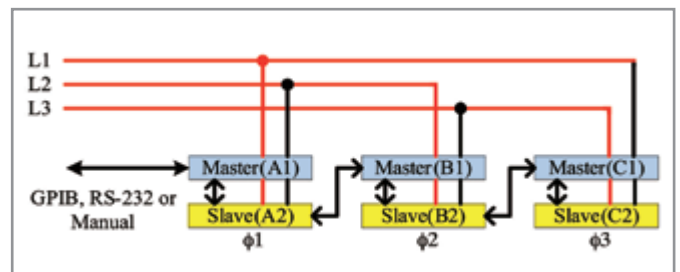
图12: 并联三相Δ接法
