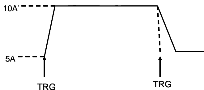
图4.12 触发操作模式
