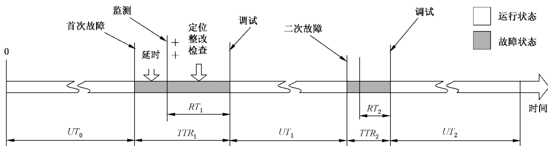
图 C.2 故障检测图解
