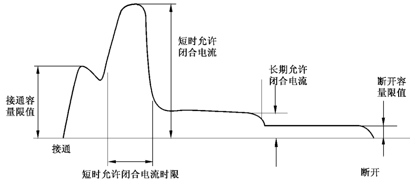
图 1 触点性能参数
