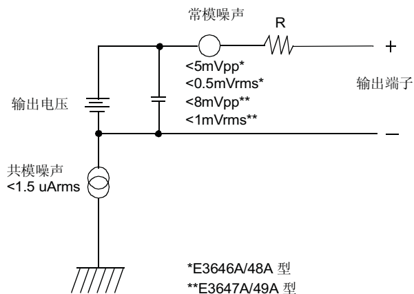
图 7-6. 共模和常模噪声源简图
