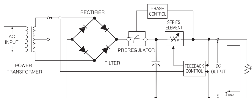
图 7-1 简单的串联电源示意图
