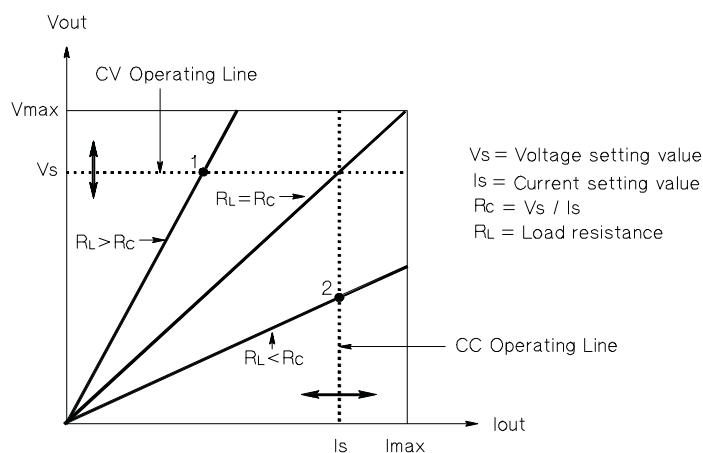
图 7-5. 输出特性
