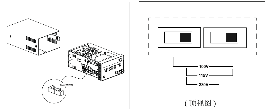
图 1-1. 线电压选择器（设置为 115 Vac）
