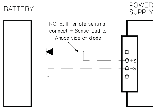
图 3-1 推荐的电池充电保护电路
