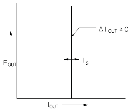
图 7-4. 理想的恒定电流电源
