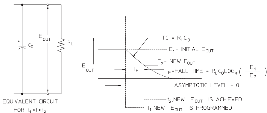
图 7-8 响应速度——电压下降编程
