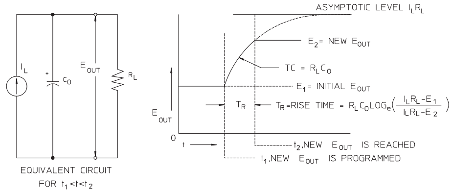
图 7-7 响应速度 —— 电压上升编程（满载）
