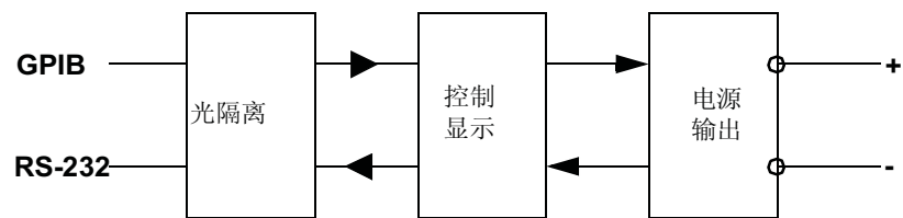
图 7-2. 示意光隔离的电源简图
