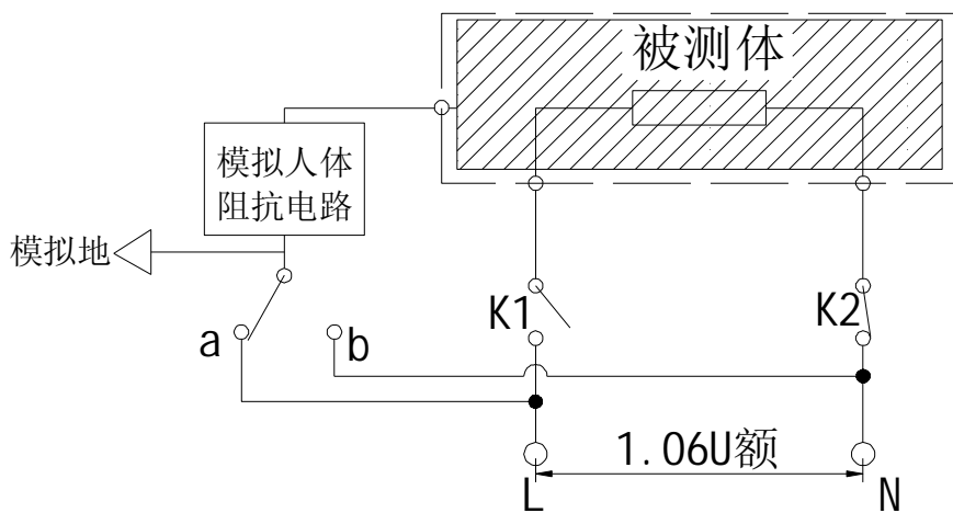
图 C-5-2 静态泄漏第二步
