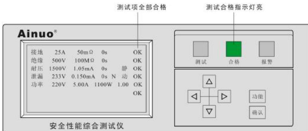
图 4-5-2 测试项全合格
