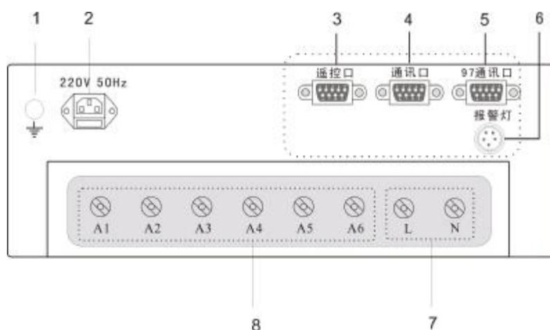
图 2-4-1 后面板示意图
