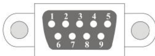
图 5-5-1 97 通讯口插座
