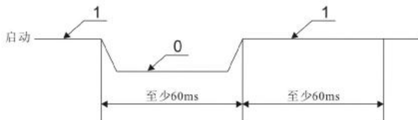
图 5-2-2 启动时序
