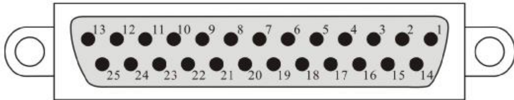
图 5-6-1 打印口插座
