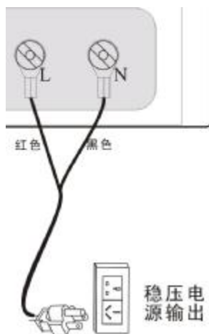
图 4-1-2 连接被测体工作电源图
