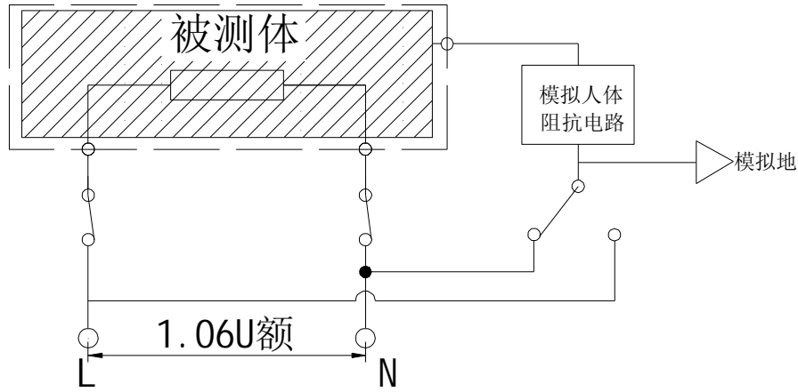
图 C-5-3 动态泄漏第一步
