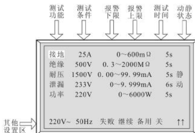
图 4-4-2 测试组设置界面
