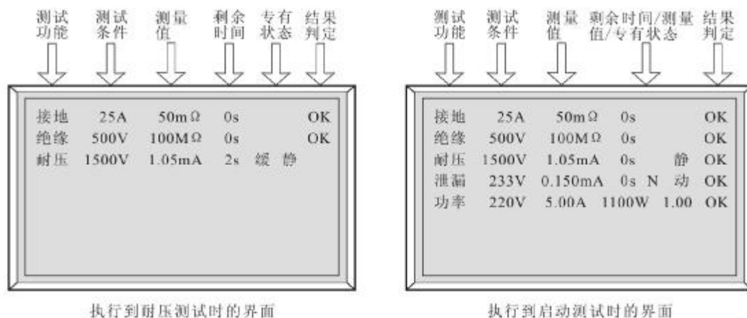
图 4-5-1 测试执行界面和指示灯
