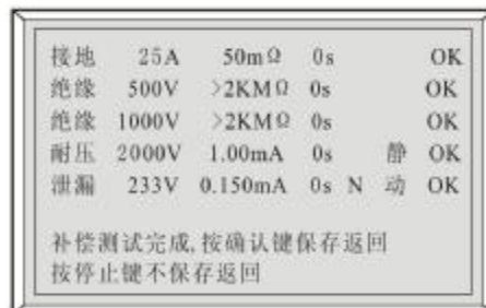
(b) 补偿测试结果
