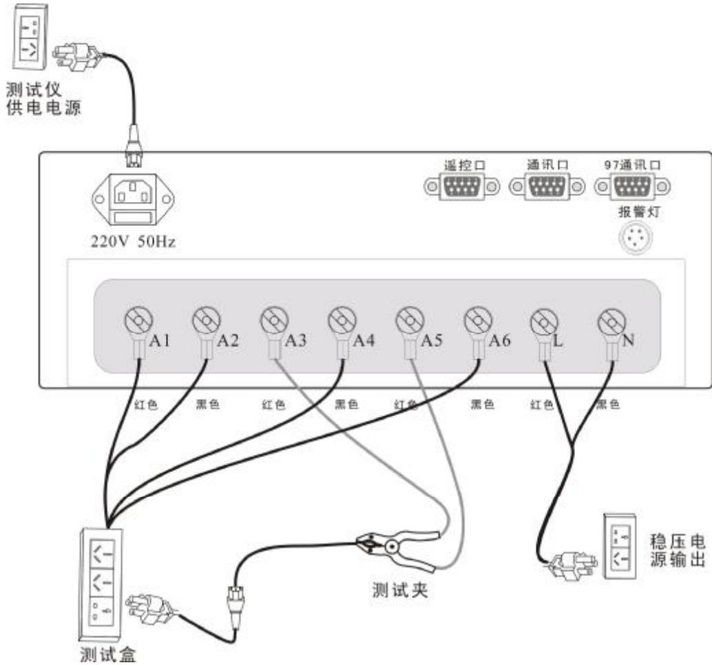
图 4-6-1 补偿测试接线示意图
