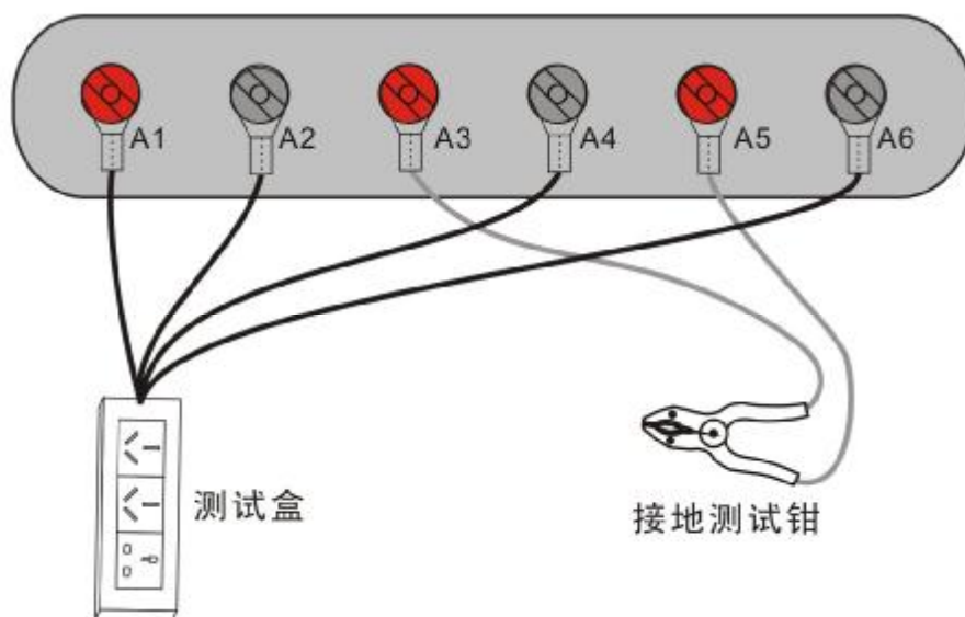
图 4-1-1 连接测试盒和接地测试钳
