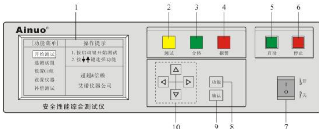
图 2-3-1 前面板示意图
