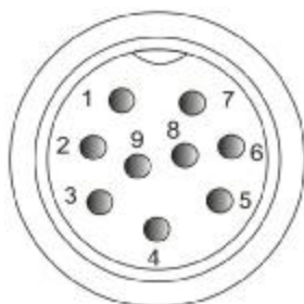
图 5-3-1 开关量接口
