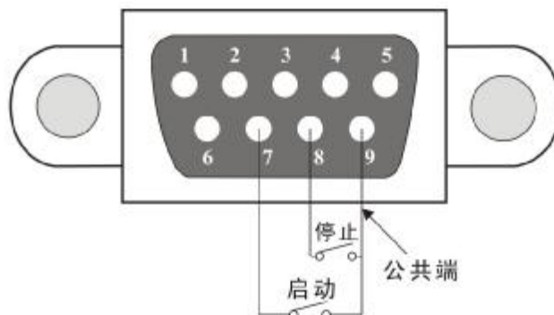
图 5-2-1 遥控口
