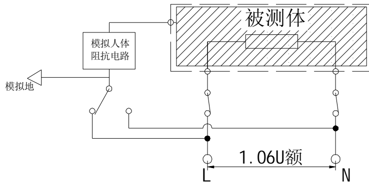
图 C-5-4 动态泄漏第二步
