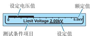
限制电压值 设定中的例
