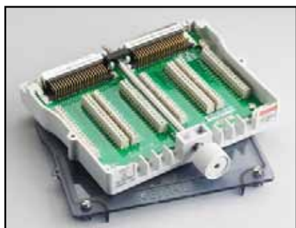
Model 3732-ST-C: 螺丝端子块。可以使用螺丝端子接入，其他矩阵尺寸包括：四口 4×28 (1W)，双口 4×28 (2W)，单口 4×56 (2W)，双口 4×56 (1W)，单口 4×112 (1W)。
