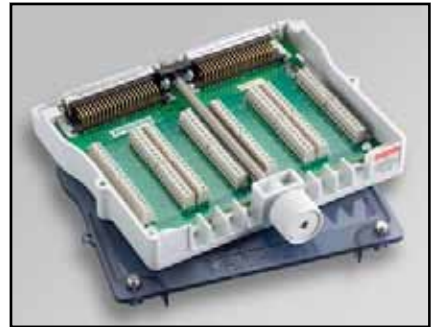
Model 3724-ST: 螺丝端子块。
