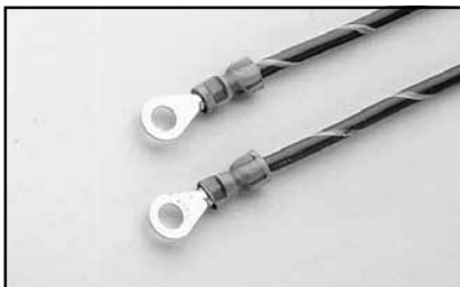
Model 8007-GND-3: 安全地线, 3m (10 英尺)。
