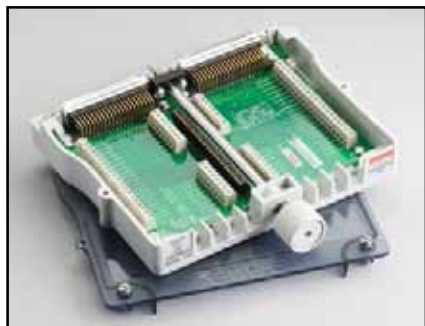
Model 3732-ST-R: 螺丝端子块。可以使用螺丝端子接入，其他矩阵尺寸包括：双口 8×28 (1W)，单口 8×28 (2W) 和单口 16×28 (1W)。
