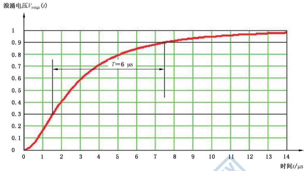
图 E.8 浪涌电压(10/700 μs): 上升时间 T
