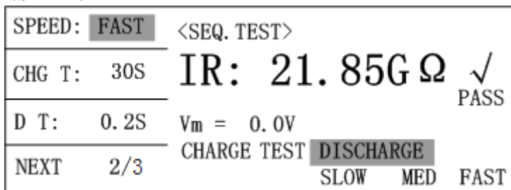
图 3-7 测试速度设定
