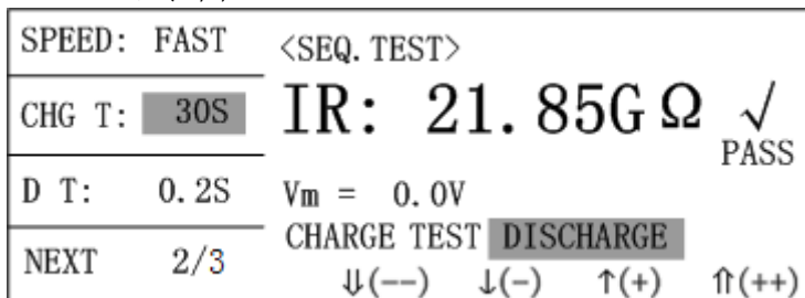
图 3-8 充电时间设定
