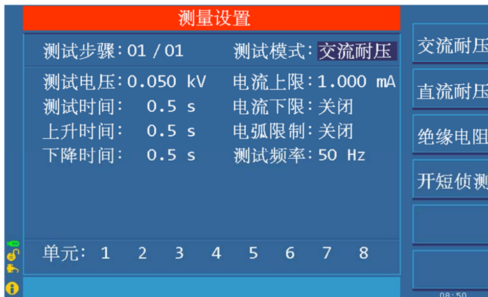
图 4.3.1 AC 设定界面示意
