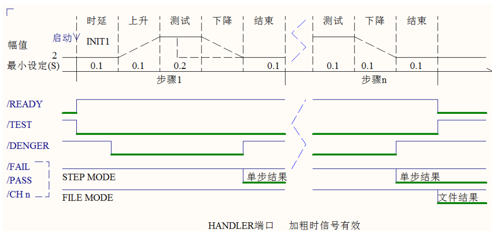
图 4.6.2: HANDLER 接口时序示意视图
