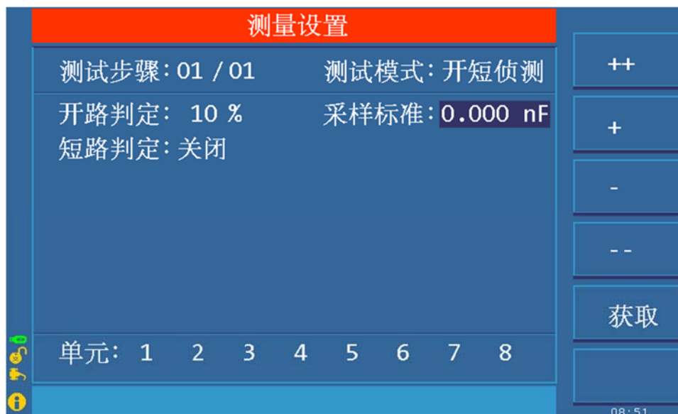
图 4.3.4 OS 设定界面示意
