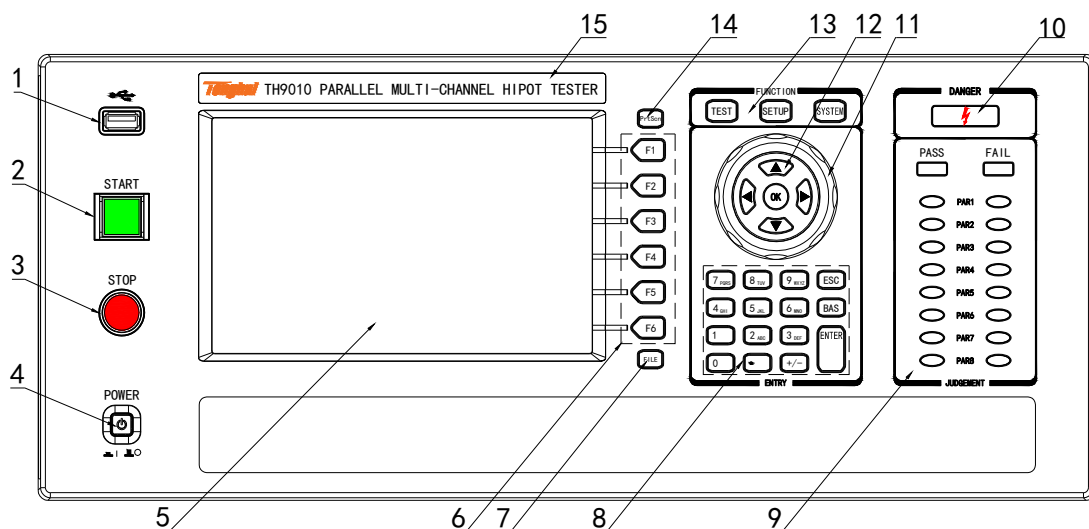
图 3-1 前面板说明
