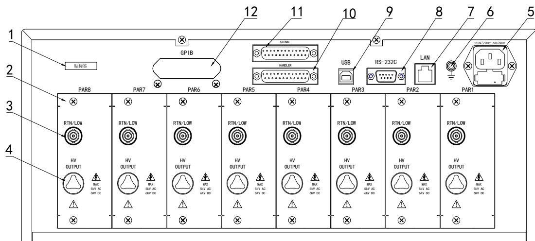
图 3-2 后面板说明
