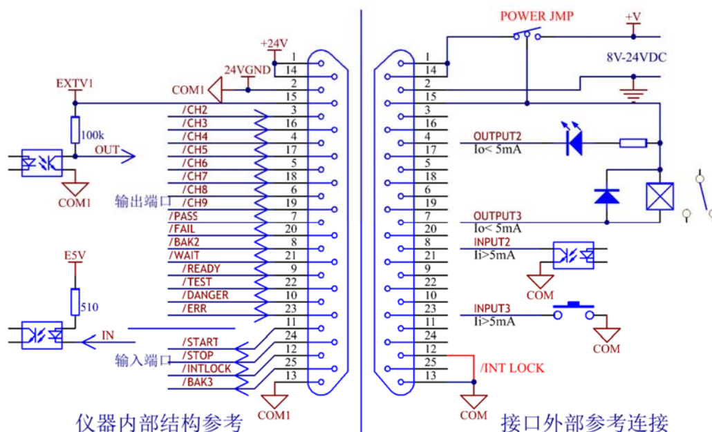
4.5.1: HANDLER 接口结构
