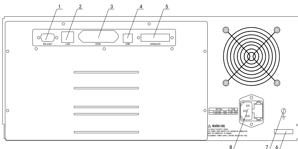
图 2-2. 后面板说明
