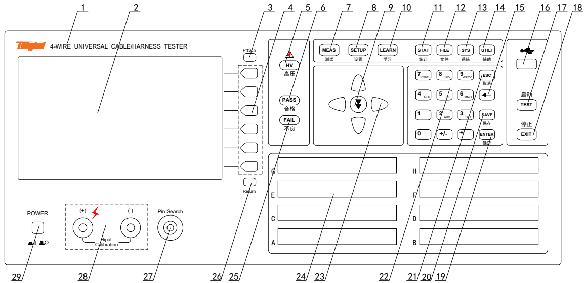
图 2-1. 前面板说明
