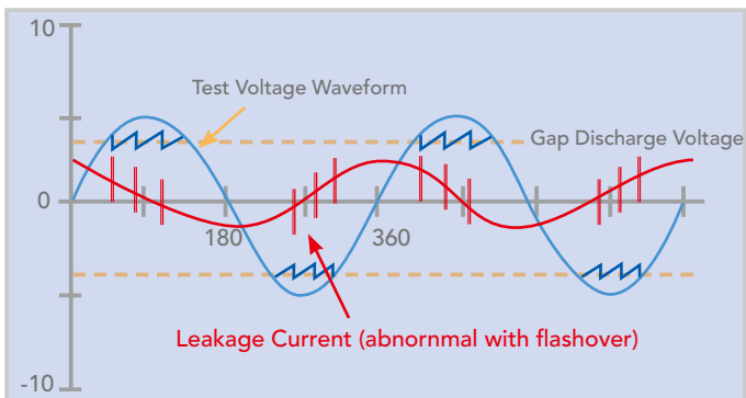
图 2：Flashover发生时高频放电电流波形
