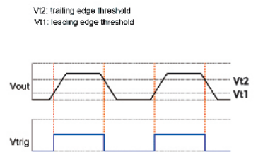
电压触发时序图
