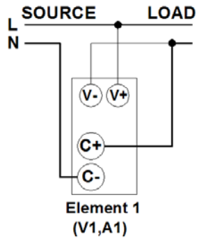
接线图1：不带传感器 单相 2 线制 (1P2W)
