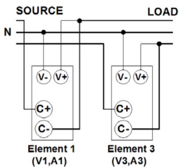
单相 3 线制 (1P3W)
