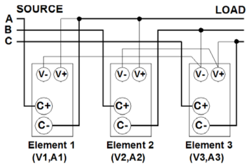
3 电压 3 电流 (3V3A)
