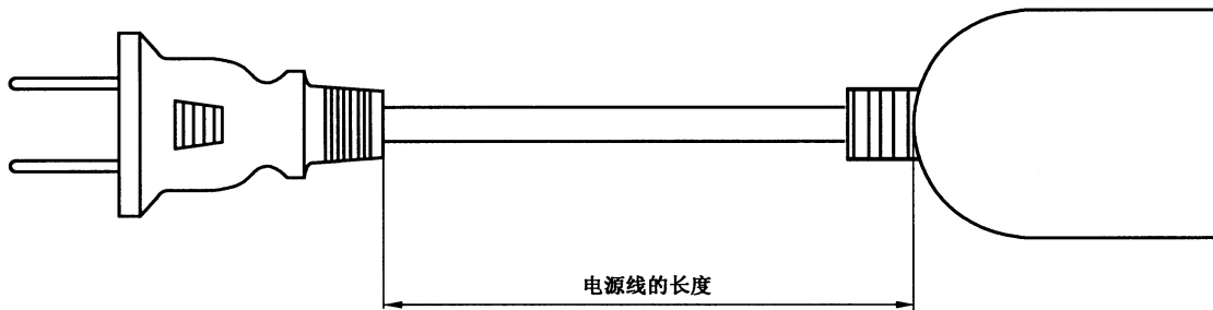
图 2 电源线长度的测量
