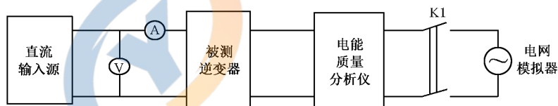
图 2 性能指标试验参考平台
