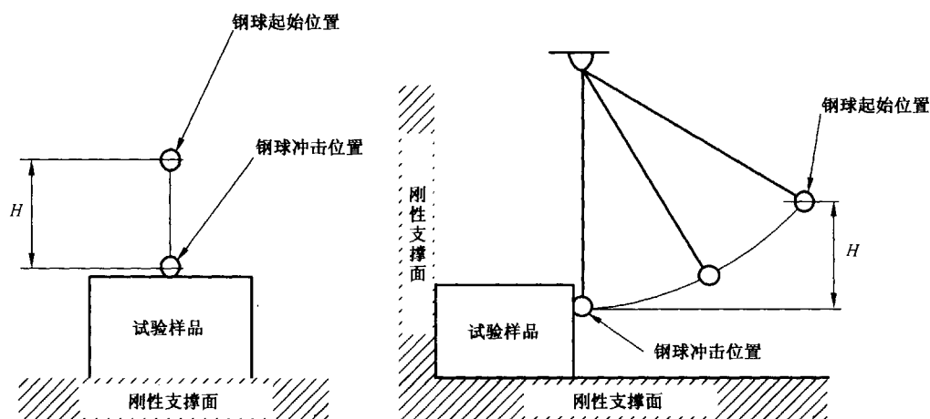
图 4A 钢球冲击试验
