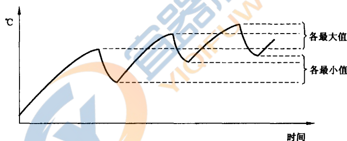
图 B.1 算术平均温度值的确定
