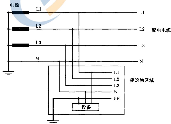
图 V.5 三相线加中线的 TT 配电系统示例
