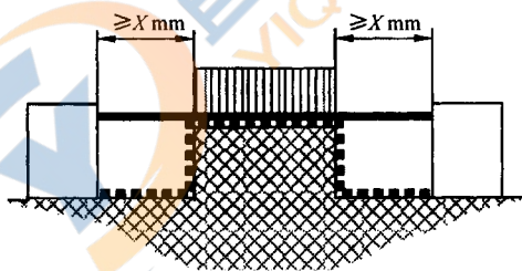
图 F.5 带窄沟槽的未粘合接缝
