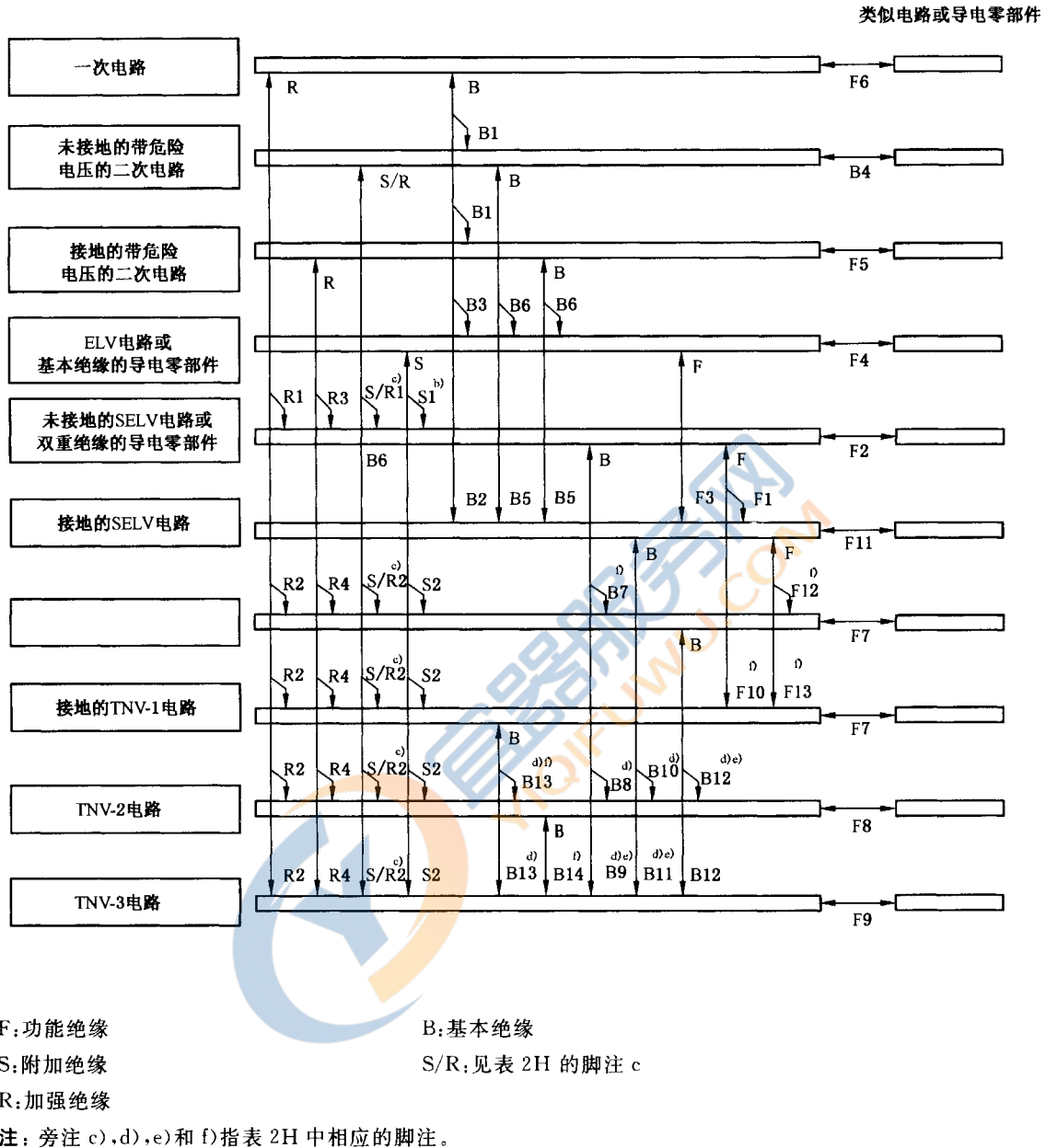
图 2H 绝缘应用示例
