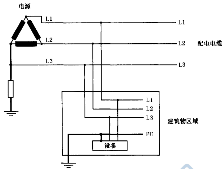
图 V.8 三相线 IT 配电系统示例
