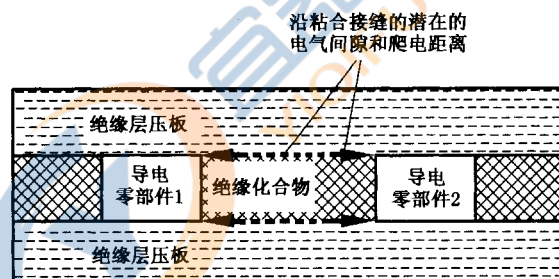
图 F.15 薄层绝缘材料
