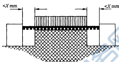
图 F.4 肋条
