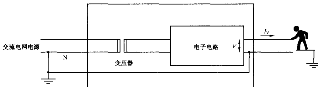
图 W.2 接地电路的接触电流
