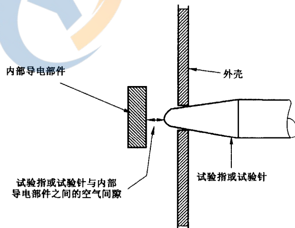
图 2C 试验探头
