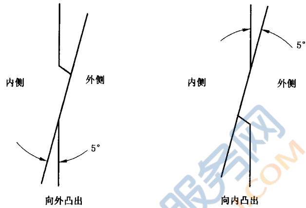
图 4C 百叶窗设计示例
