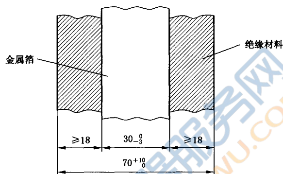
图 AA. 4 金属箔在绝缘材料上的位置
