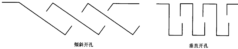
图 4B 防止垂直进入的开孔截面设计示例
