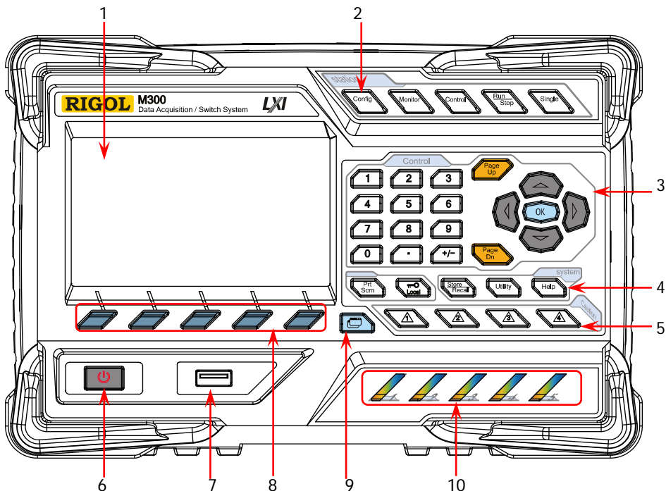
图 1-3 M300 前面板
