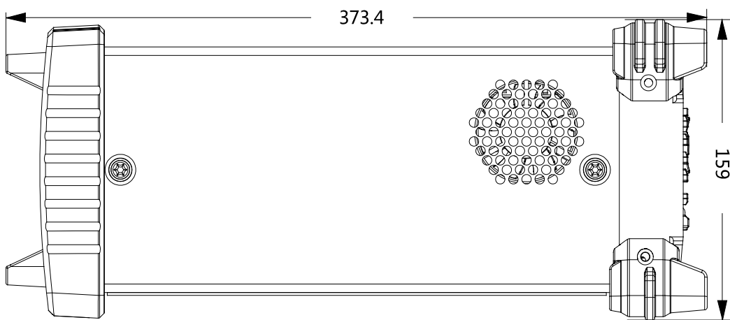
图 1-2 侧视图
