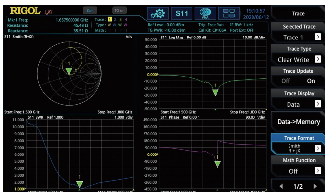
VNA模式可以实现对元器件、电路网络的S11、S21以及故障点定位的测量，通过史密斯圆图、极坐标等多种显示更精确地表征被测件的网路特性
