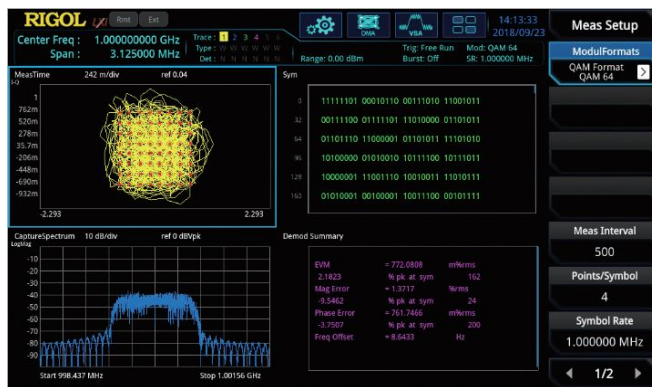
用户可以进行自由设置测量显示结果，一次性呈现信号多种视图并通过灵活的布局调整获得更清晰显示
