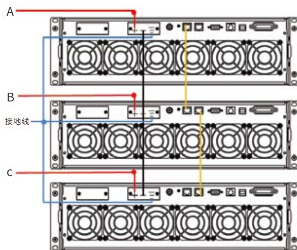
三角形接法
