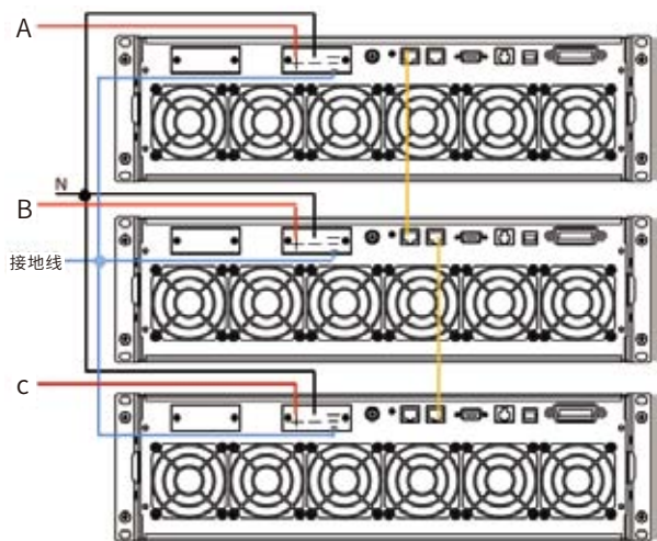
星形接法
