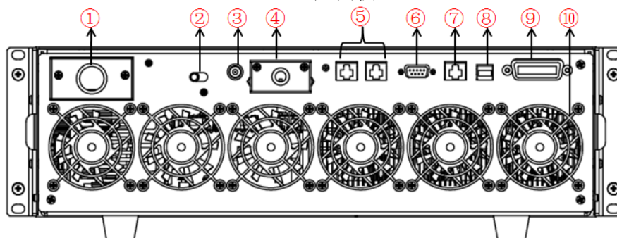
IT7322/IT7322H/IT7324/IT7324H 后面板
