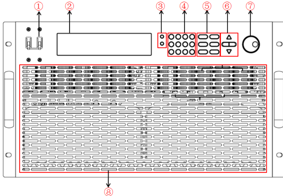
IT7326H 前面板
