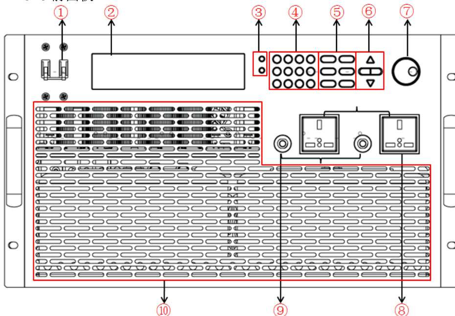
IT7326 前面板
