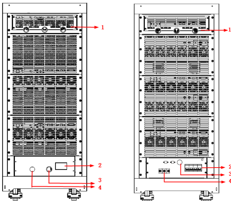
IT7324HT 后面板图示
