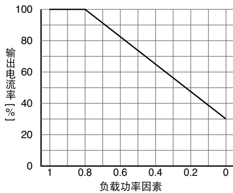
■ 负载功率因素—额定输出电流特性
