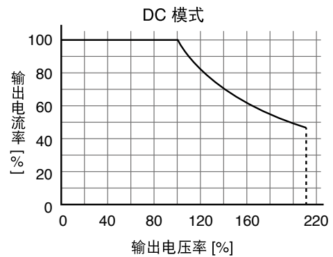
■ 输出电压率—额定输出电流特性 (DC 模式)
