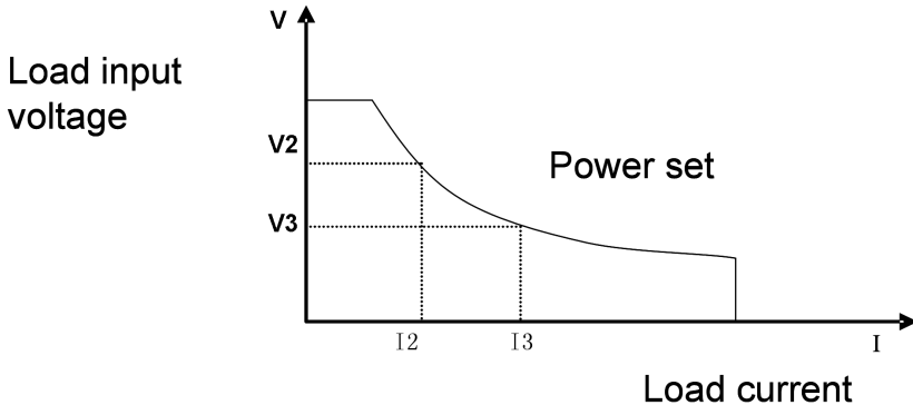
图 4.9 定功率模式
