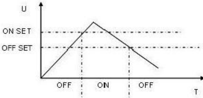
图 4.2 加载卸载模式
