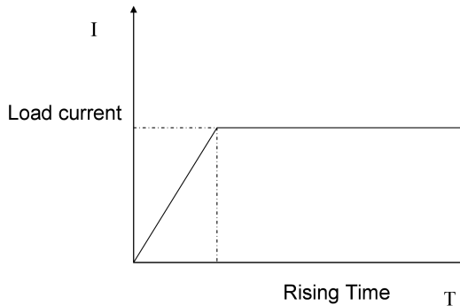
图 4.3 软启动电流模式
