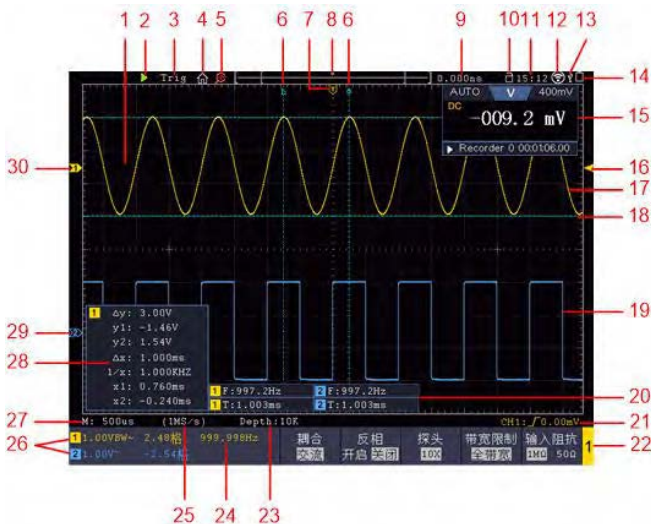
图 3- 5：显示界面说明图
