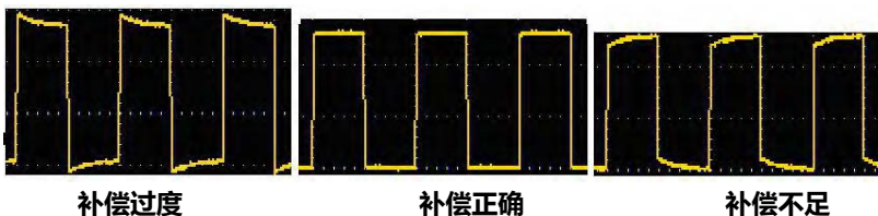
图 3- 7：探头补偿显示波形
