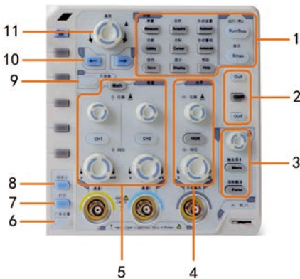
图 3- 4：按键和旋钮控制区说明图
