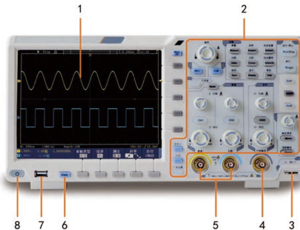
图 3- 1：示波器前面板
