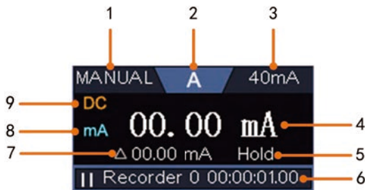
图 5- 3 : 万用表显示窗
