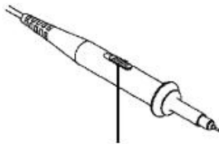
图 3- 9 : 探头衰减开关
