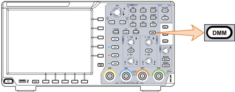
图 5- 2 : 万用表按键
