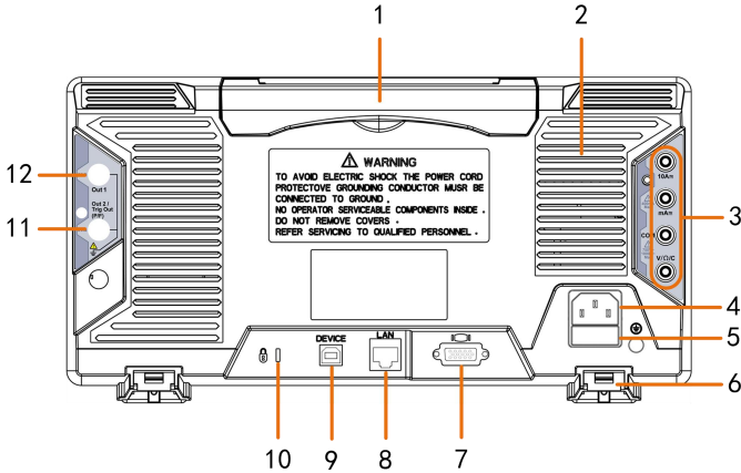
图 3- 2：示波器后面板
