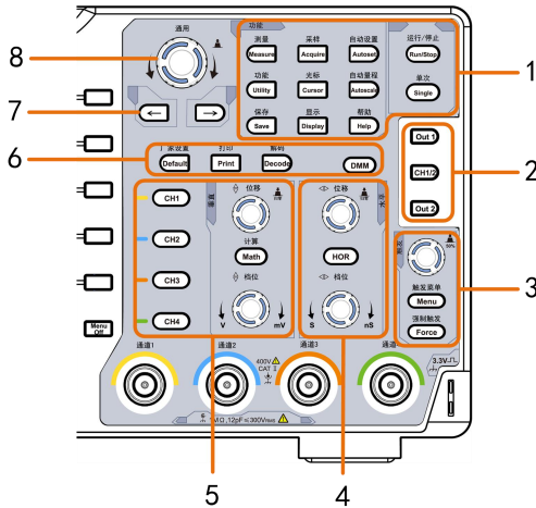
图 3- 3：按键和旋钮控制区说明图
