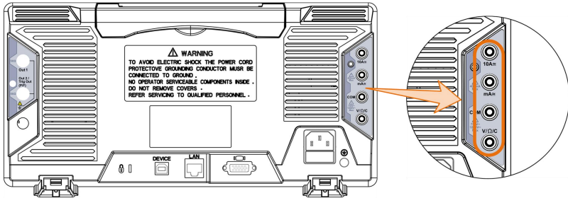
图 5- 1：万用表输入端
