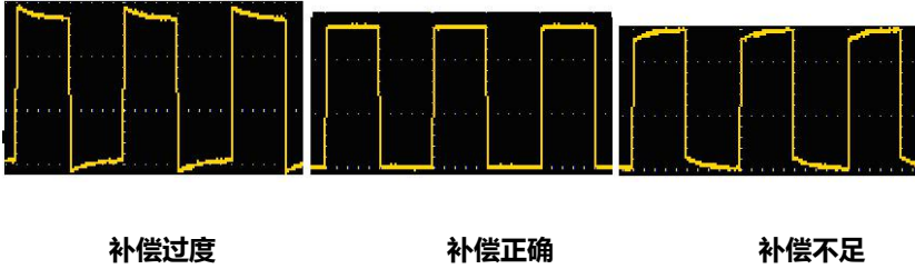
图 3- 6：探头补偿显示波形
