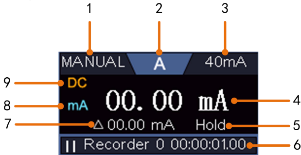
图 5- 3 : 万用表显示窗
