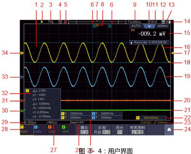
图 3-4：用户界面
