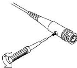
图 7- 3 : 探头调整
