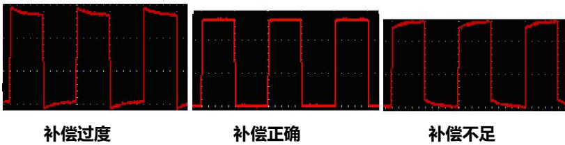
图 7- 2 : 探头补偿显示波形
