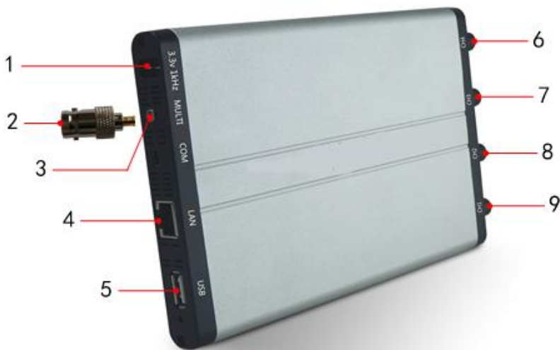
图 3- 1 : 示波器接口
