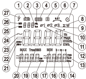
图3 LCD全显图
