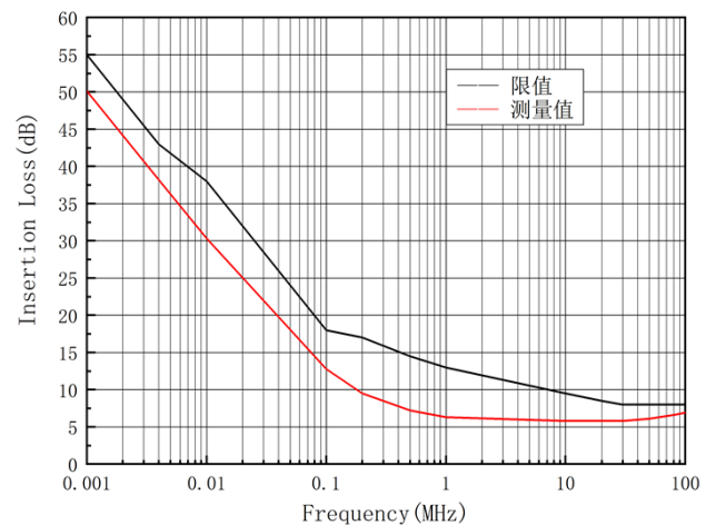
BCIP7637-3 电流注入钳插入损耗曲线
