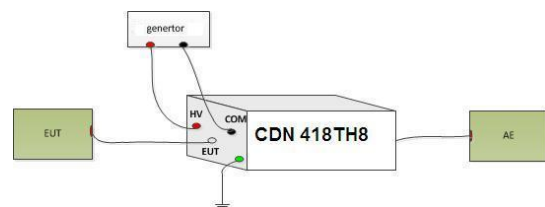
设计原理图:
