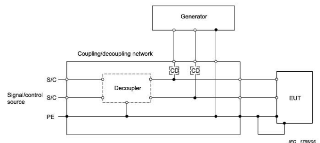
设计原理图:
