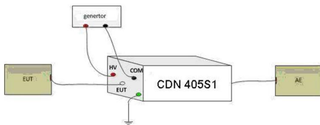
标准原理图 1 (屏蔽线两端接地):
