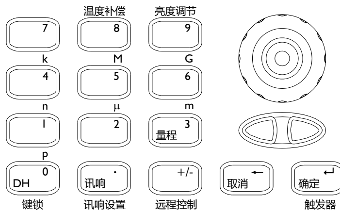
图 3-3 键区二
