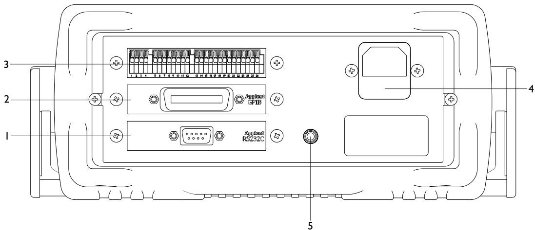
图 3-5 后面板
