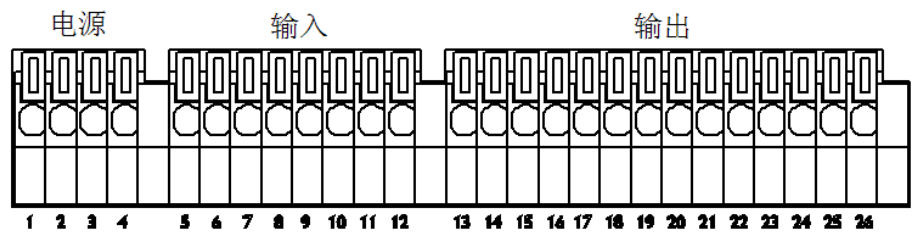
图 5-1 接线端子
