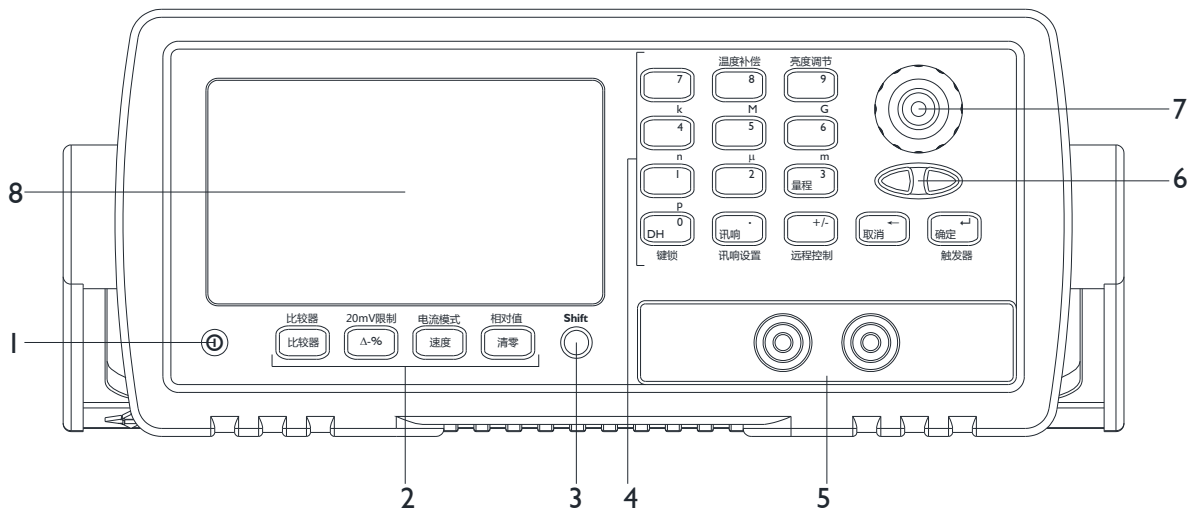
图 3-1 前面板
