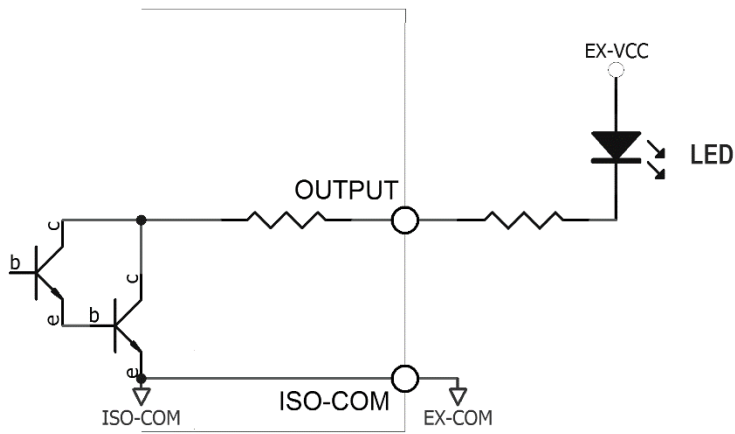
图 10-9 控制发光二极管或光电耦合器
