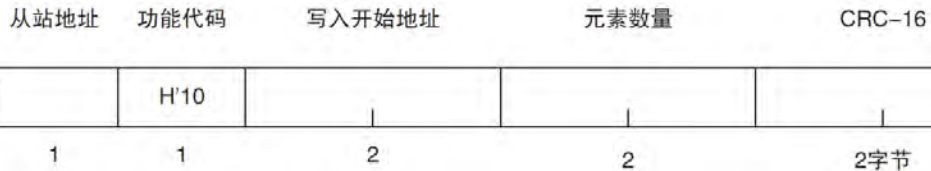
图 13-8 写入多个寄存器 (0x03) 响应帧
