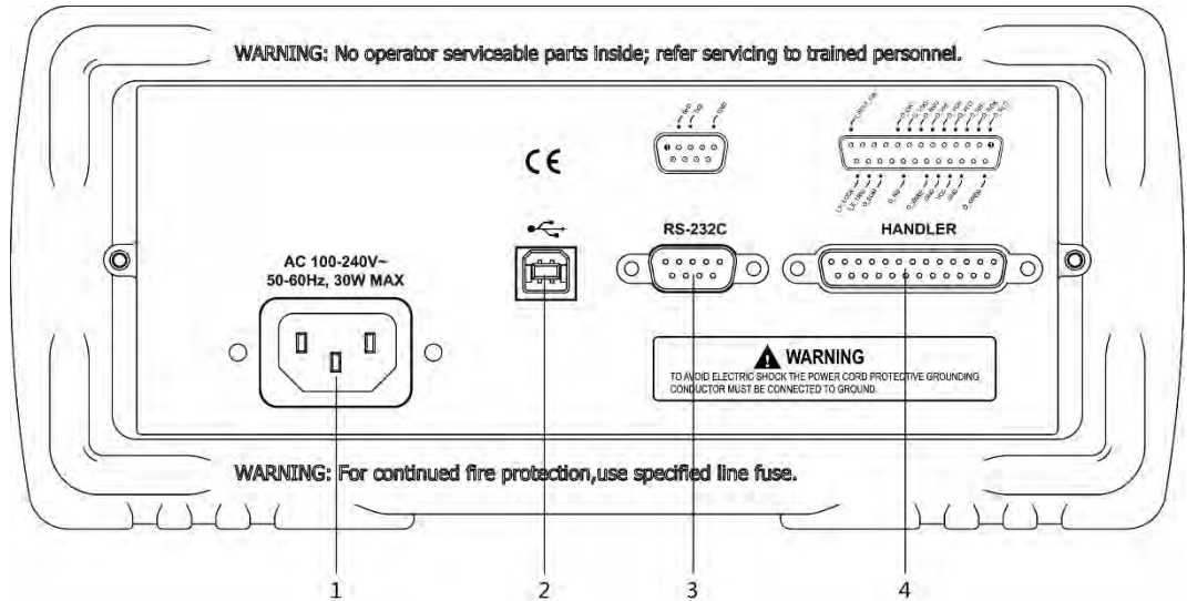
图 3-2 后面板
