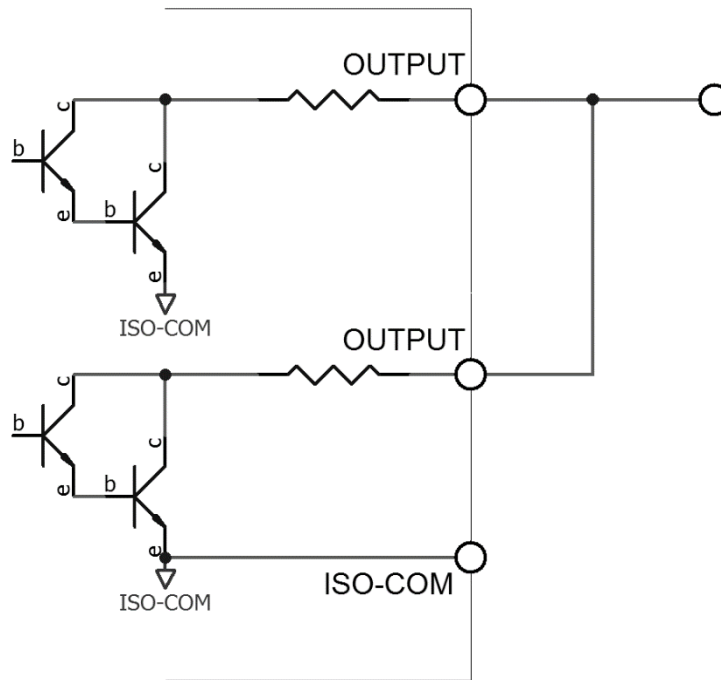
图 10-11 双端口输出组成逻辑或电路
