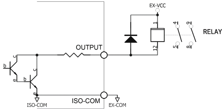
图 10-8 控制继电器
