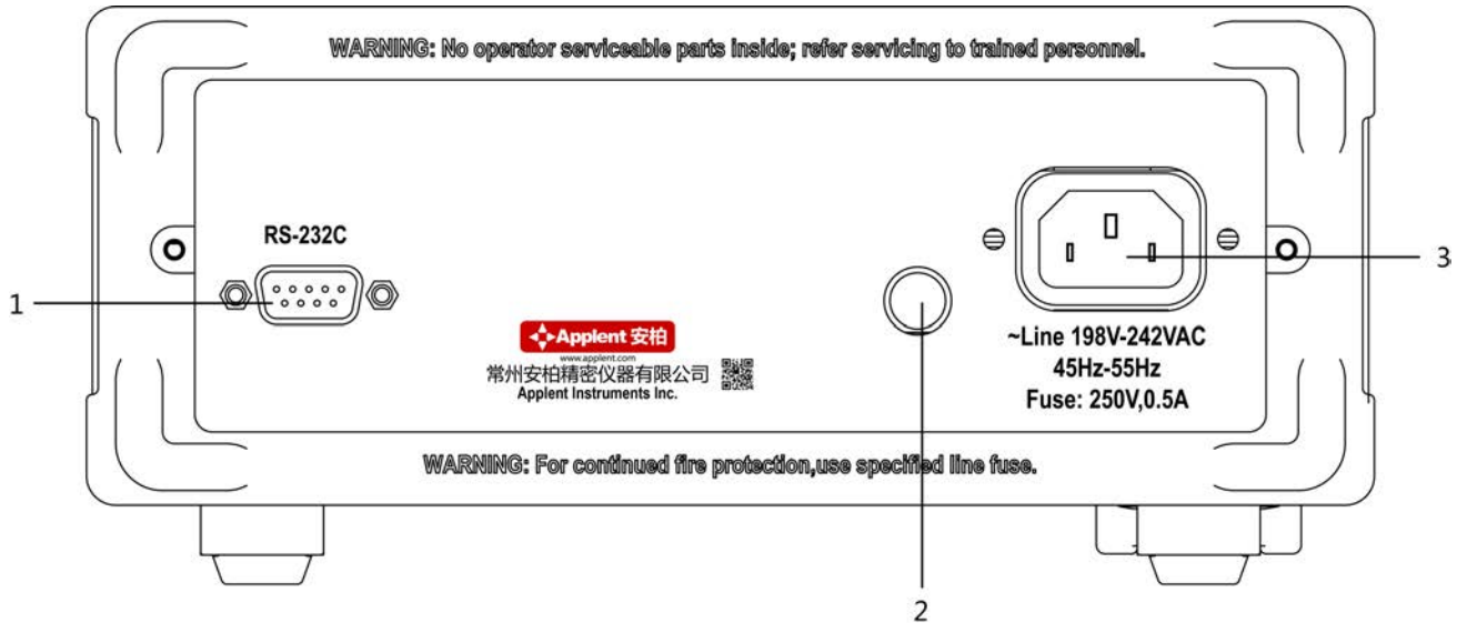
图 3-2 后面板图
