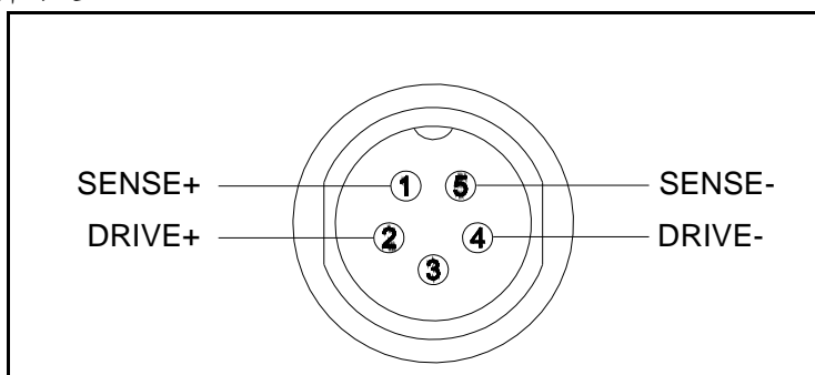
图 3-3 测试端引脚的定义
