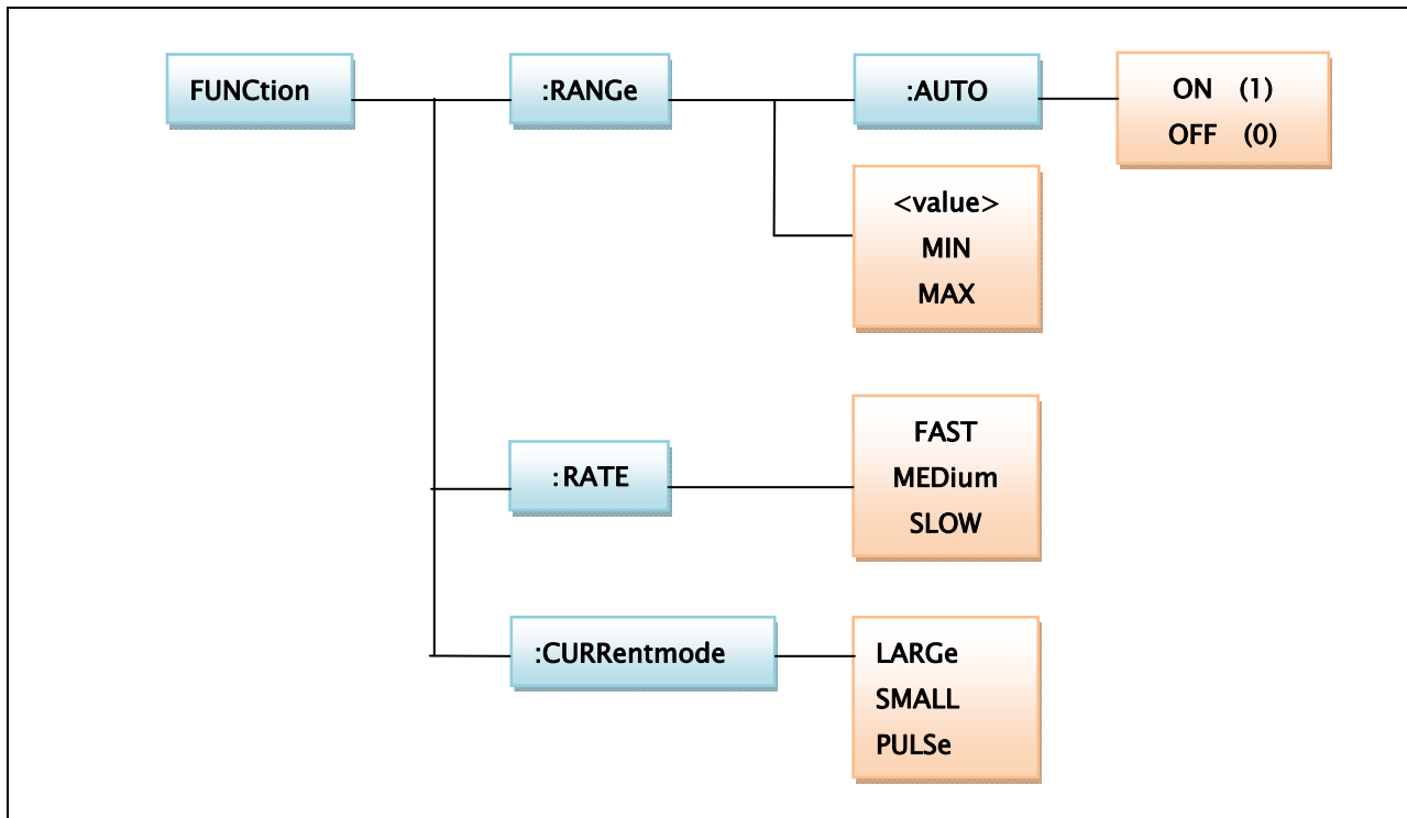
FUNCTION 指令系统树
