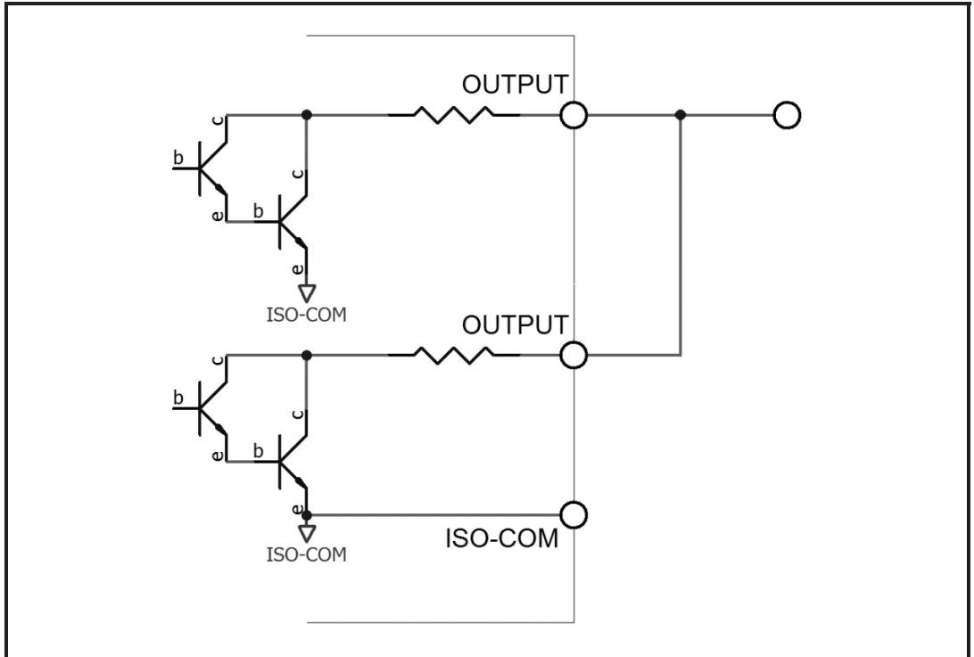
图 7-12 输出到 PLC 负公共端子
