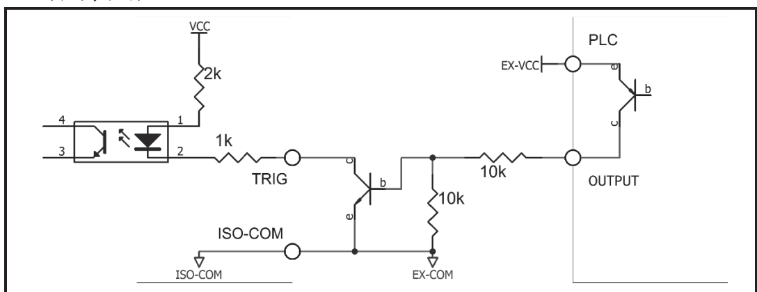
图 7-7 使用 PLC 正公共端子控制
