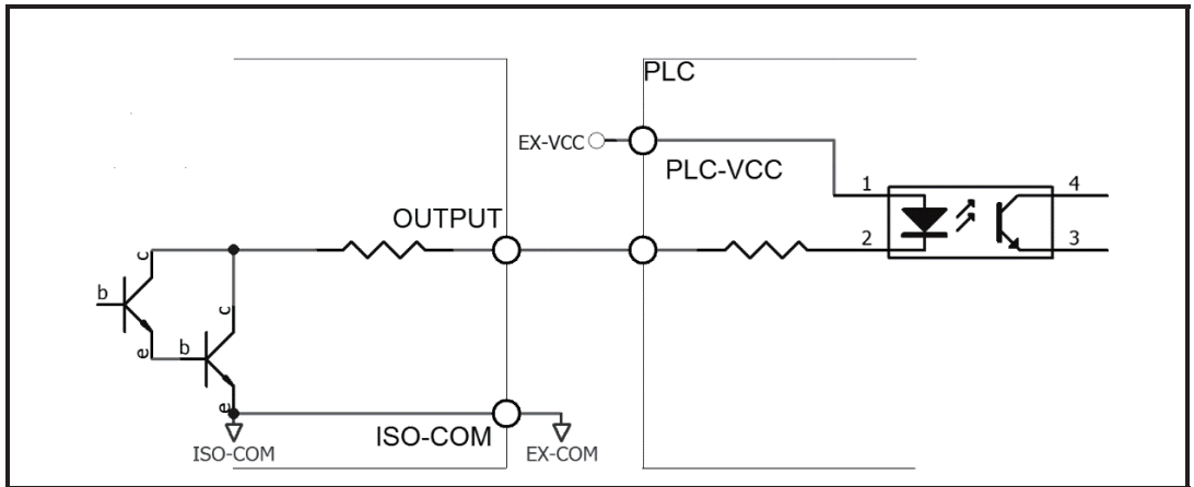
图 7-12 输出到 PLC 负公共端子
