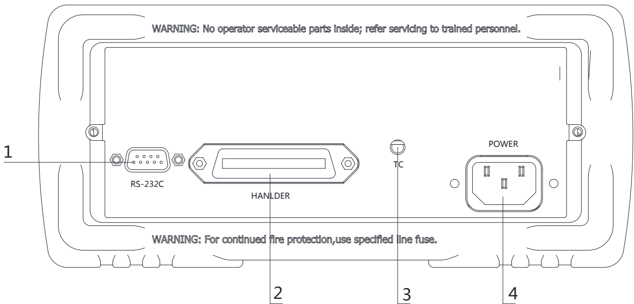
图 3-2 后面板
