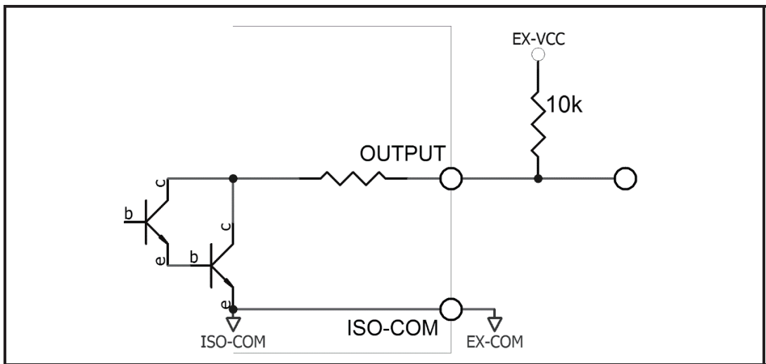
图 7-11 双端口输出组成逻辑或电路
