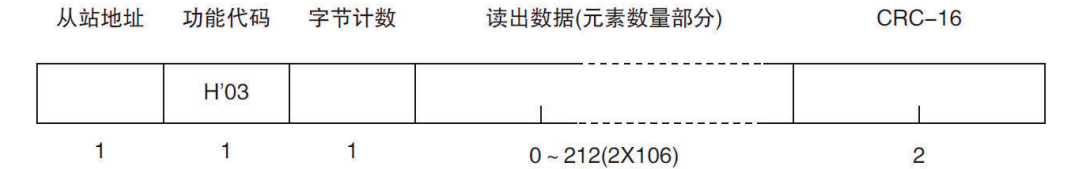
图 10-6 读出多个寄存器 (0x03) 响应帧
