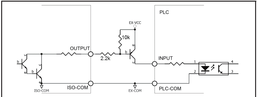
图 7-13 输出到 PLC 正公共端子
