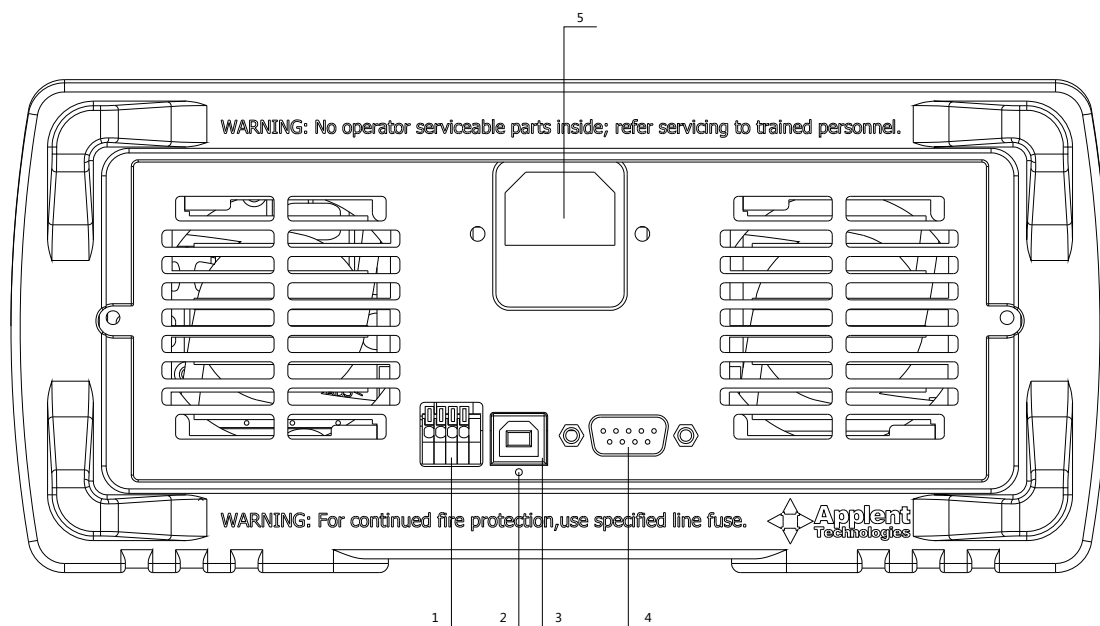
图 3-5 后面板
