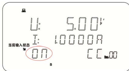
图 3-10 负载输入状态
