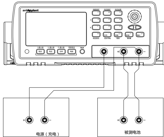
图 3-9 电池寿命测试的连接方法
