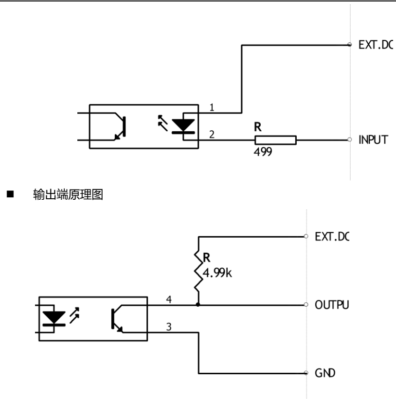
图 5-2 内部原理图
