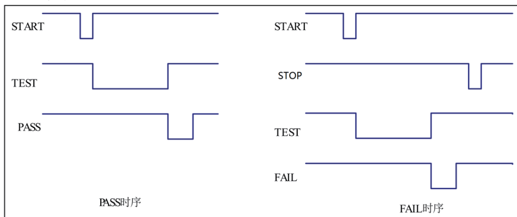
图 8-5 PLC 时序图
