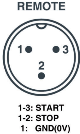
图 8-2 遥控接口插座（公）
