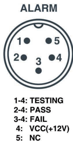
图 8-1 报警灯接口插座（公）
