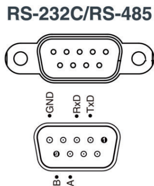
图 8-3 通讯接口（管脚定义参见“9.1.1 RS232C 连接”）
