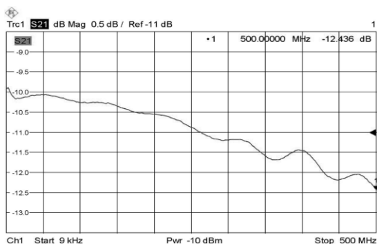
图 1 频响曲线
