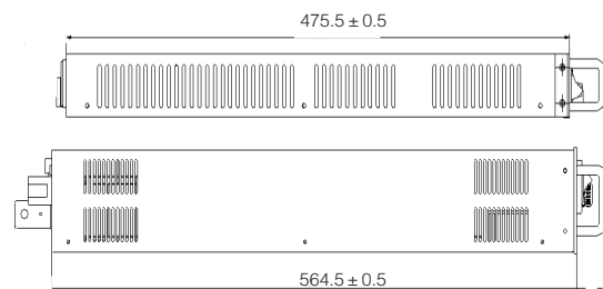
侧视图
