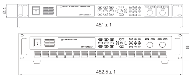
正视图
