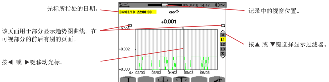
图91: 不包含MIN-AVG-MAX的 \cos \phi(L1)
