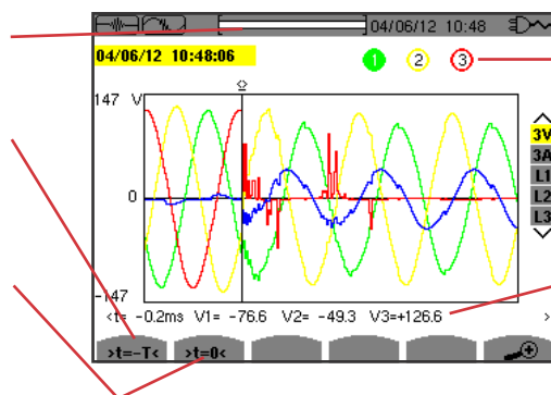
图 40: 曲线图形式显示三相五线连接暂态测量实例
