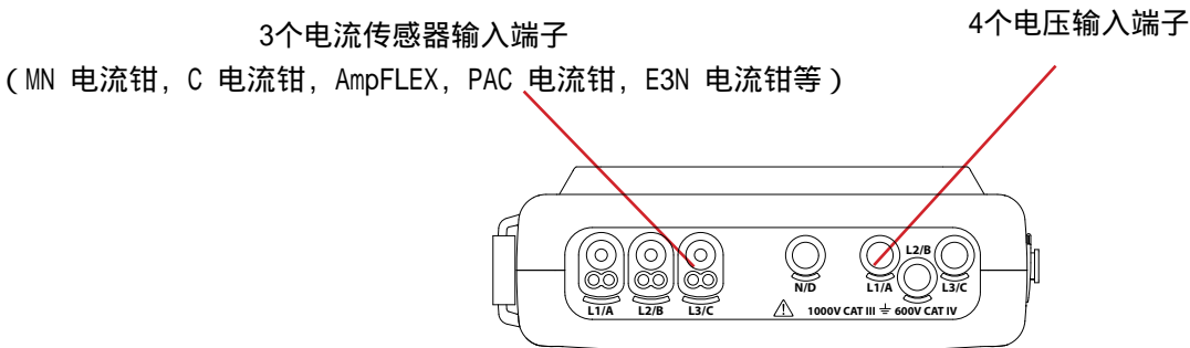
图4：仪器接口端子
