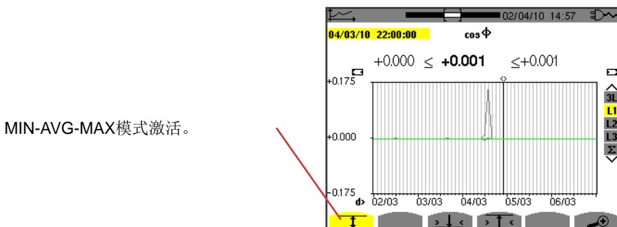
图92: 含MIN-AVG-MAX的 \cos \phi(L1)
