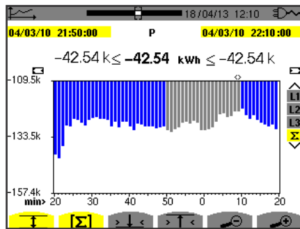
图90: 含MIN-AVG-MAX的 Ph(\Sigma)
