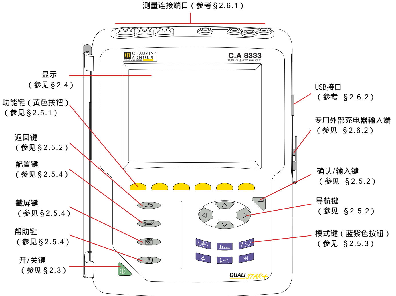
图2：仪器全览
