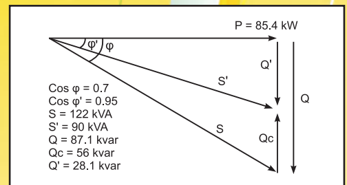
通过增加无功功率 Q_c ，将 PF 由 0.7 增加到 0.95
