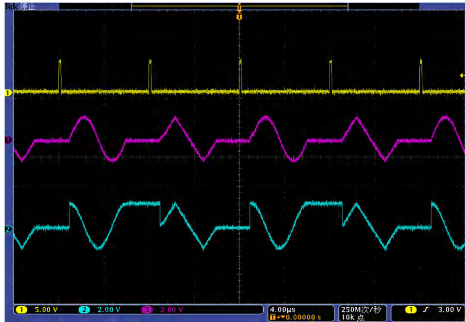
图 4.31 任意波触发示意图（波形段 单次）
