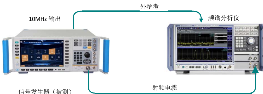
图 8.6 小功率测试
