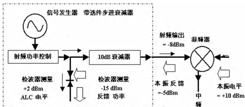
图 4.14 反向功率影响，-8dBm 耦合输出
