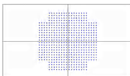
图 2.10 512QAM
