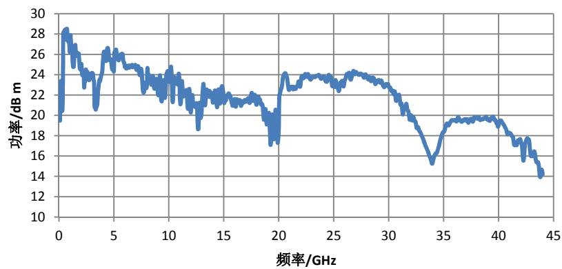
1465F-V最大输出功率（选件H05）
