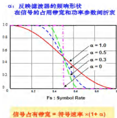
附图11 信道带宽与 \alpha 之间的关系示意图
