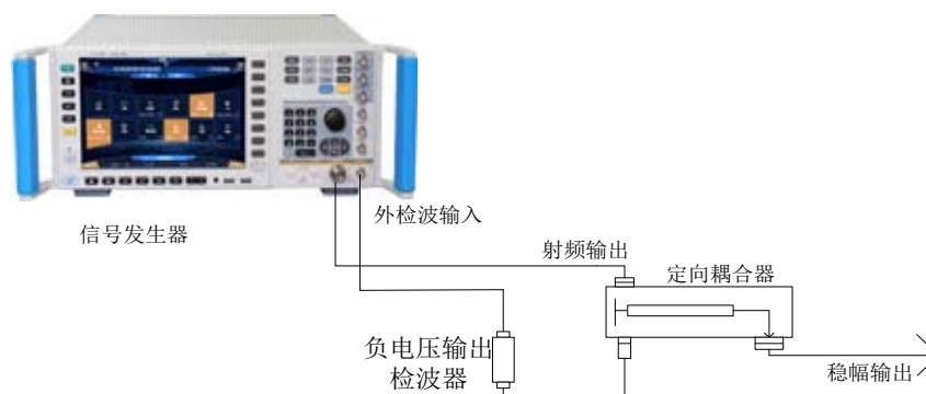
图 4.13 ALC 电路外部稳幅测量连接框图
