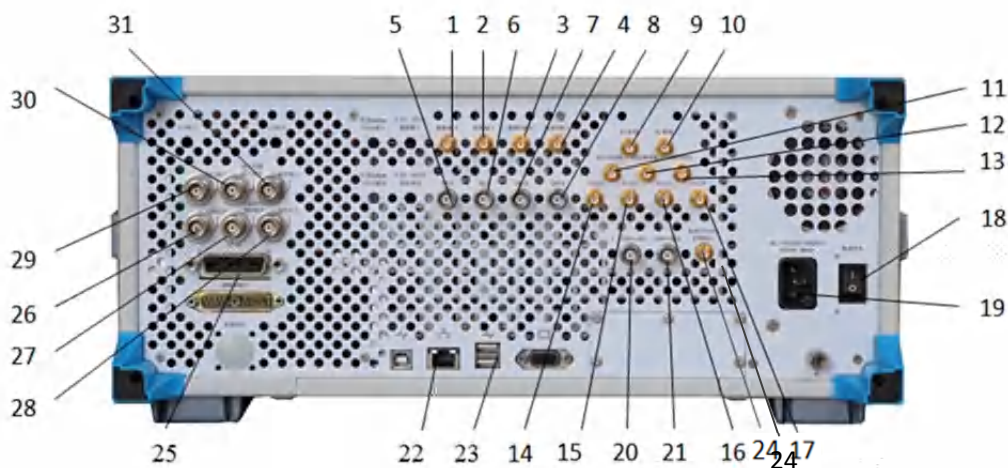
图 3.12 仪器后面板
