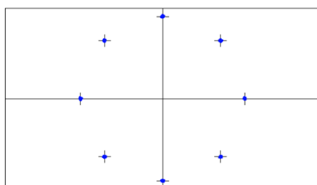
图 2.9 8PSK
