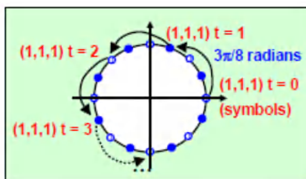
附图10 EDGE矢量图
