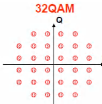
附图6 32QAM星座图
