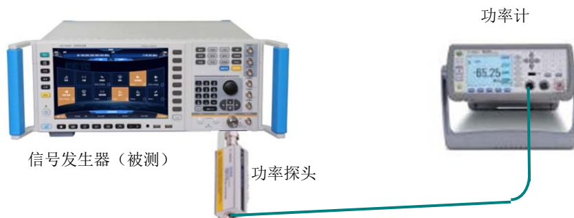
图 8.5 最大稳幅输出功率测试
