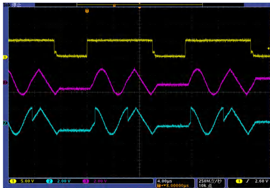
图 4.32 任意波触发示意图（门控 高有效）
