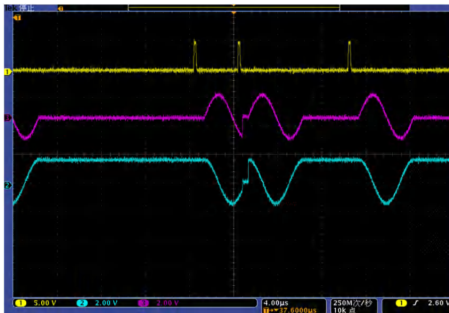
图 4.30 任意波触发示意图（单次 实时重复触发）
