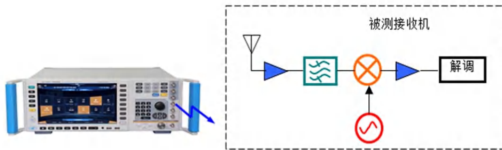
图 2.14 1465 在高性能接收机测试中的应用
