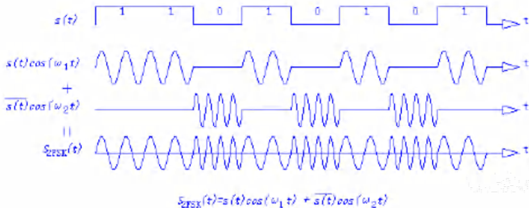
附图1 2FSK示意图
