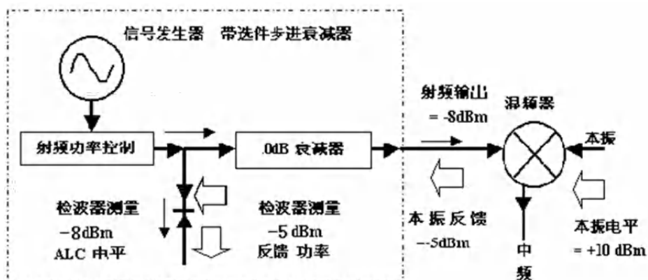
图 4.14 反向功率影响，-8dBm 耦合输出
