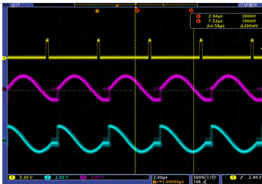
图 4.27 任意波触发示意图（连续 实时）
