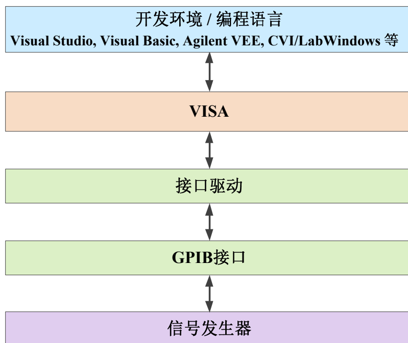
图6.6 程控软硬件层
