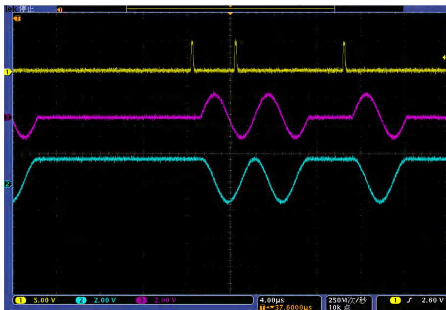
图 4.29 任意波触发示意图（单次 缓冲重复触发）
