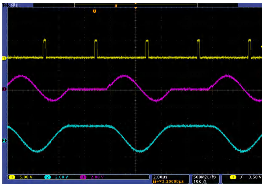
图 4.28 任意波触发示意图（单次 忽略重复触发）
