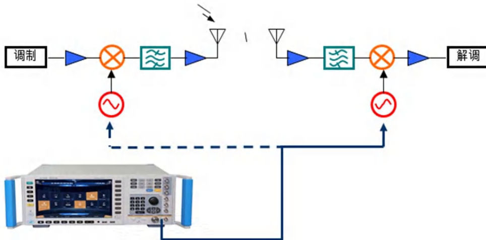
图 2.15 1465 在本振替代中的应用
