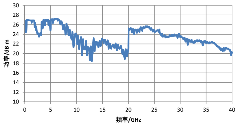
1465F最大输出功率(选件H05)
