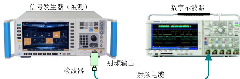
图 8.7 脉冲调制开关比测试
