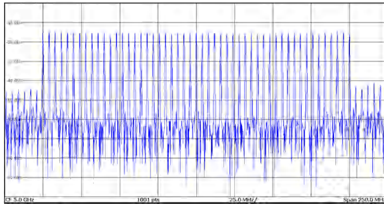
图 2.5 5GHz 载波 200MHz 调制带宽多音信号
