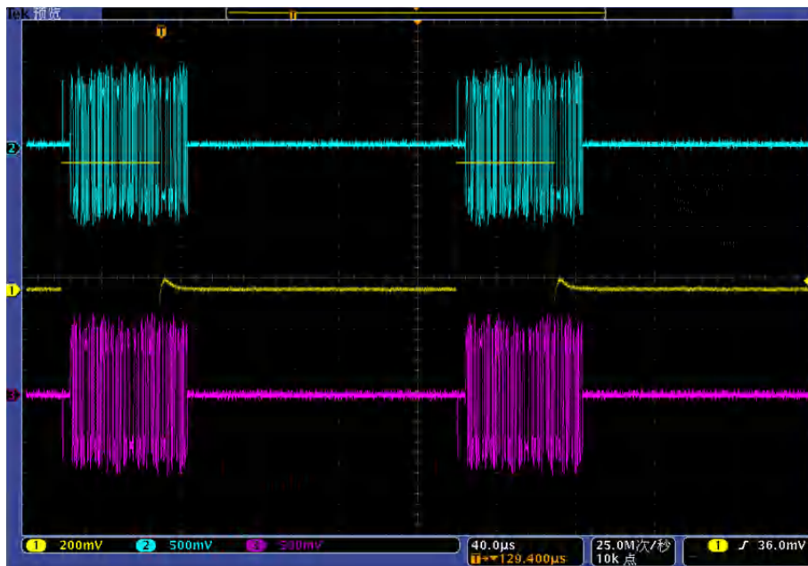
图 4.24 基带触发示意图（连续 单次）
