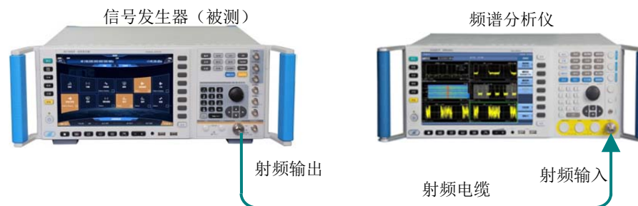
图 8.4 谐波测试
