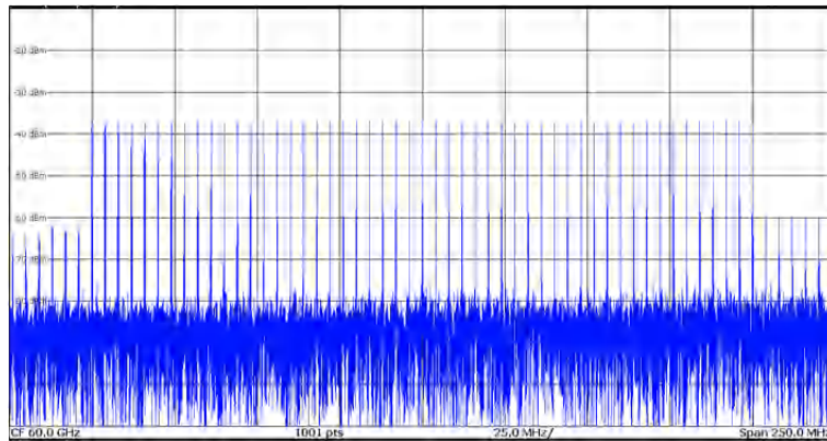
图 2.6 60GHz 载波 200MHz 调制带宽多音信号
