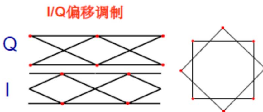
附图8 QPSK调制方式
