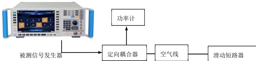
图 8.11 源驻波测试
