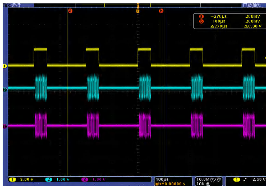
图 4.25 基带触发示意图（门控 高有效）
