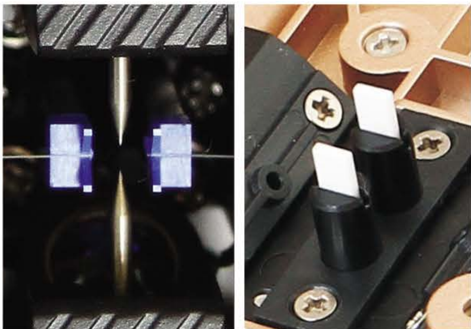
高精度陶瓷V型槽
