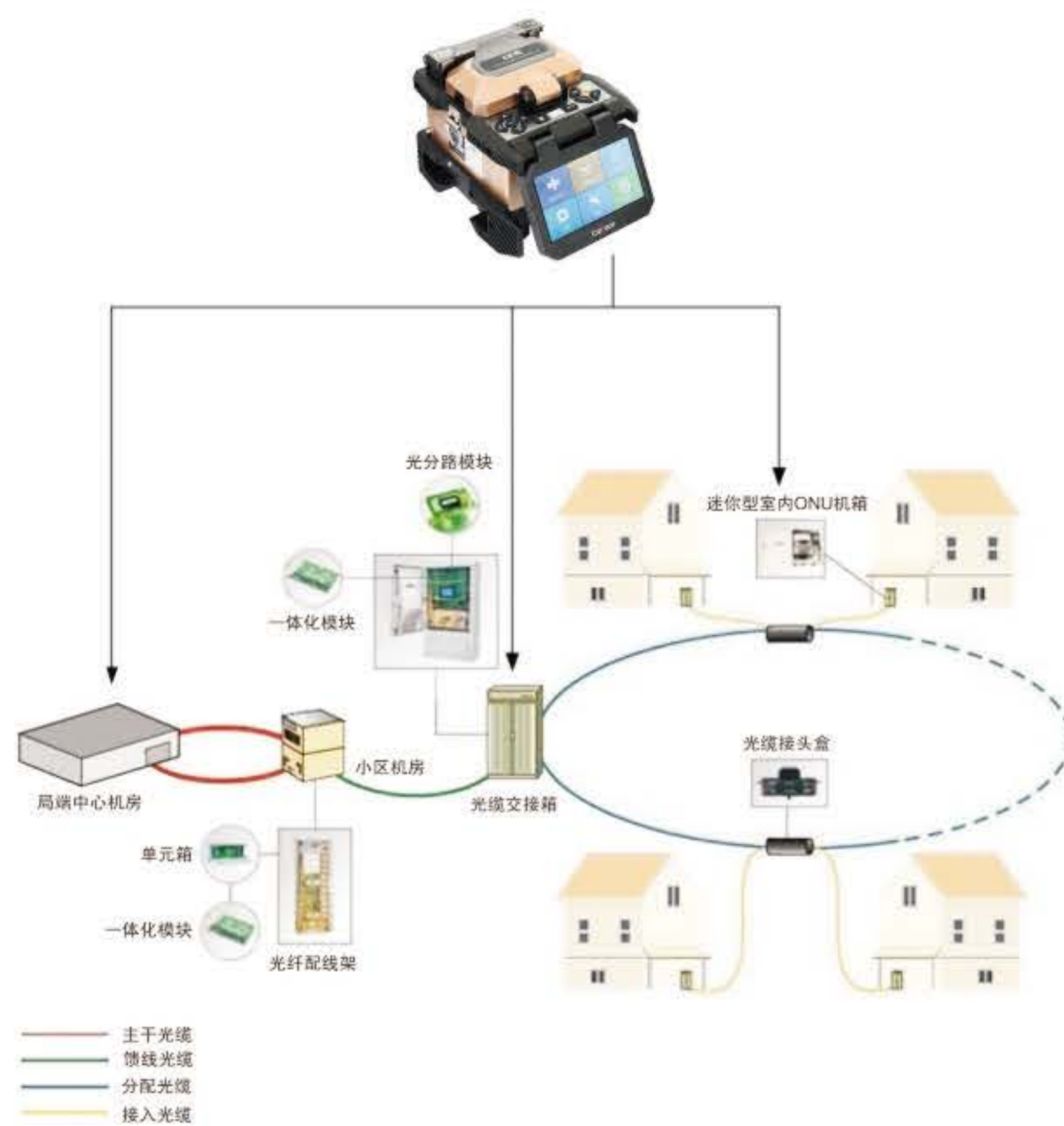
6481系列光纤熔接机典型应用
