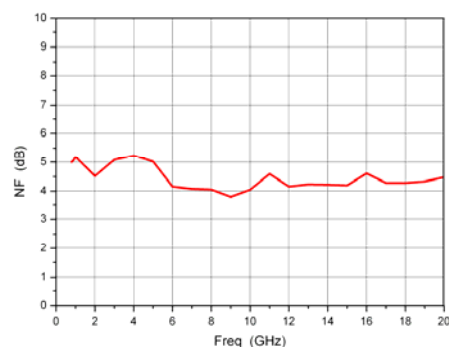
噪声系数 VS 频率
