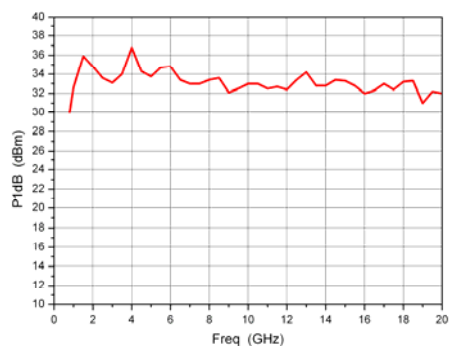
1dB 压缩输出功率 VS 频率
