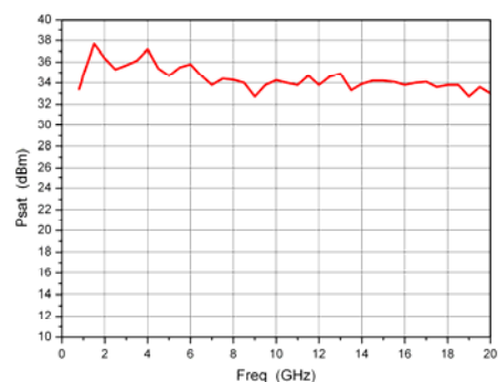
饱和输出功率 V S 频率
