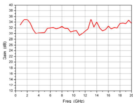
小信号增益 VS 频率
