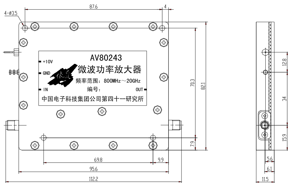
AV80243 结构尺寸 (mm)
