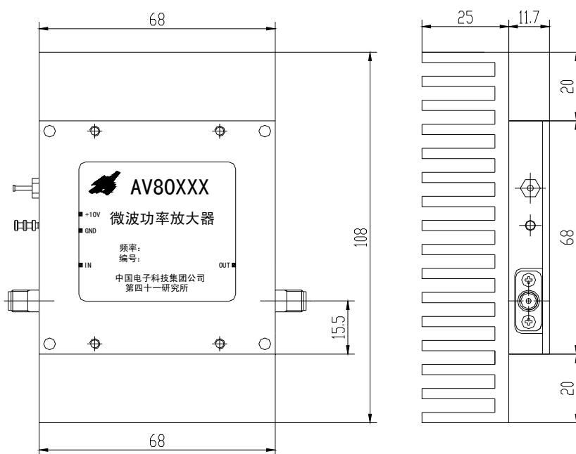
AV80259-S 结构尺寸 (单位: mm)
