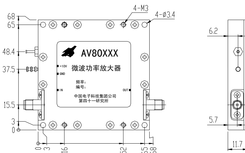
AV80259 结构尺寸 (单位: mm)
