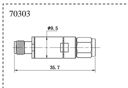
70303 结构尺寸 (mm)
