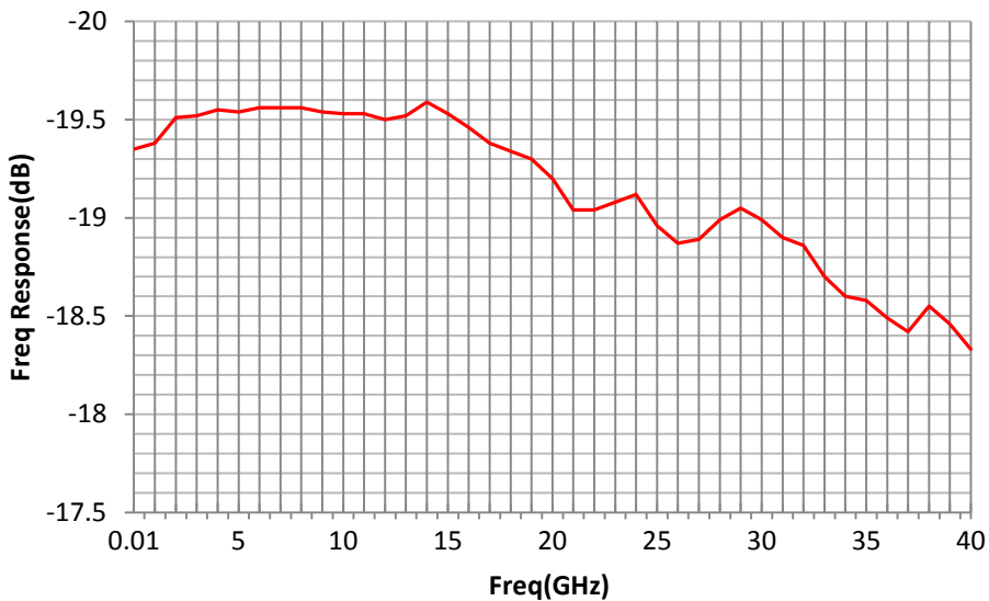
检波频响 VS 频率
