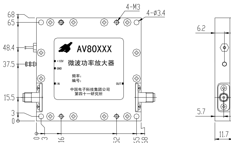
AV80262 结构尺寸 (单位: mm)
