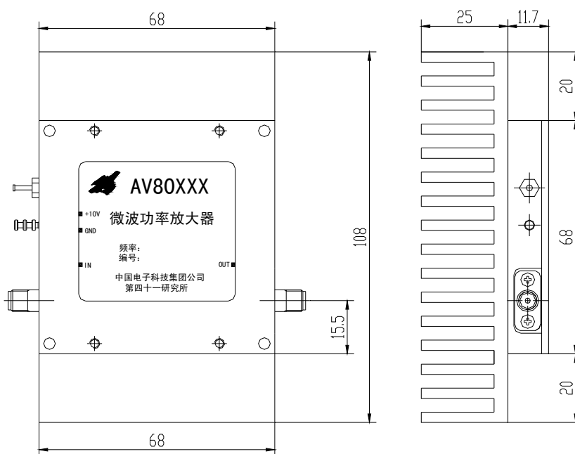
AV80262-S 结构尺寸 (单位: mm)
